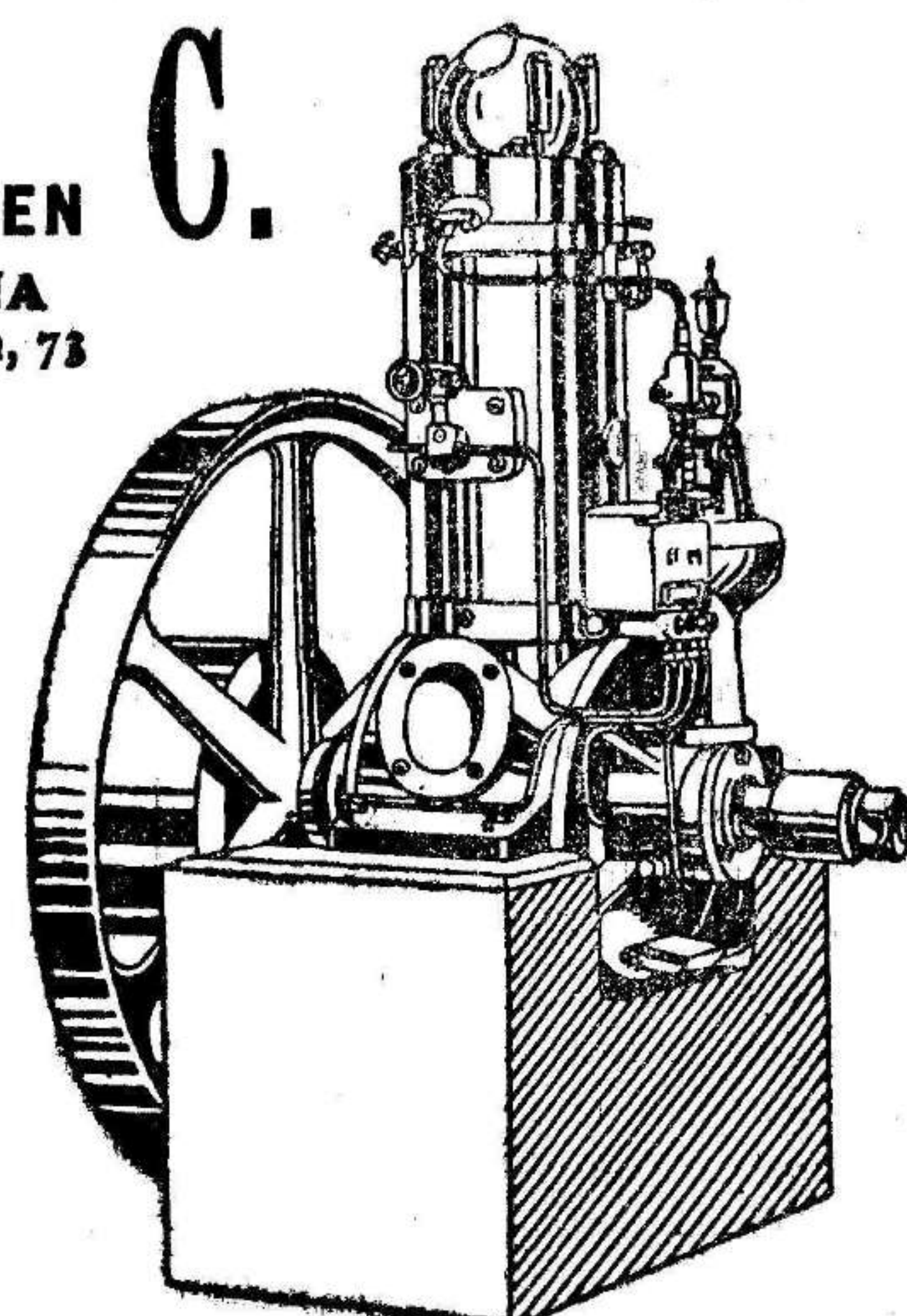
Motor para aceites pesados, sin válvulas, sin mecanismo adecuado para trilladoras.
