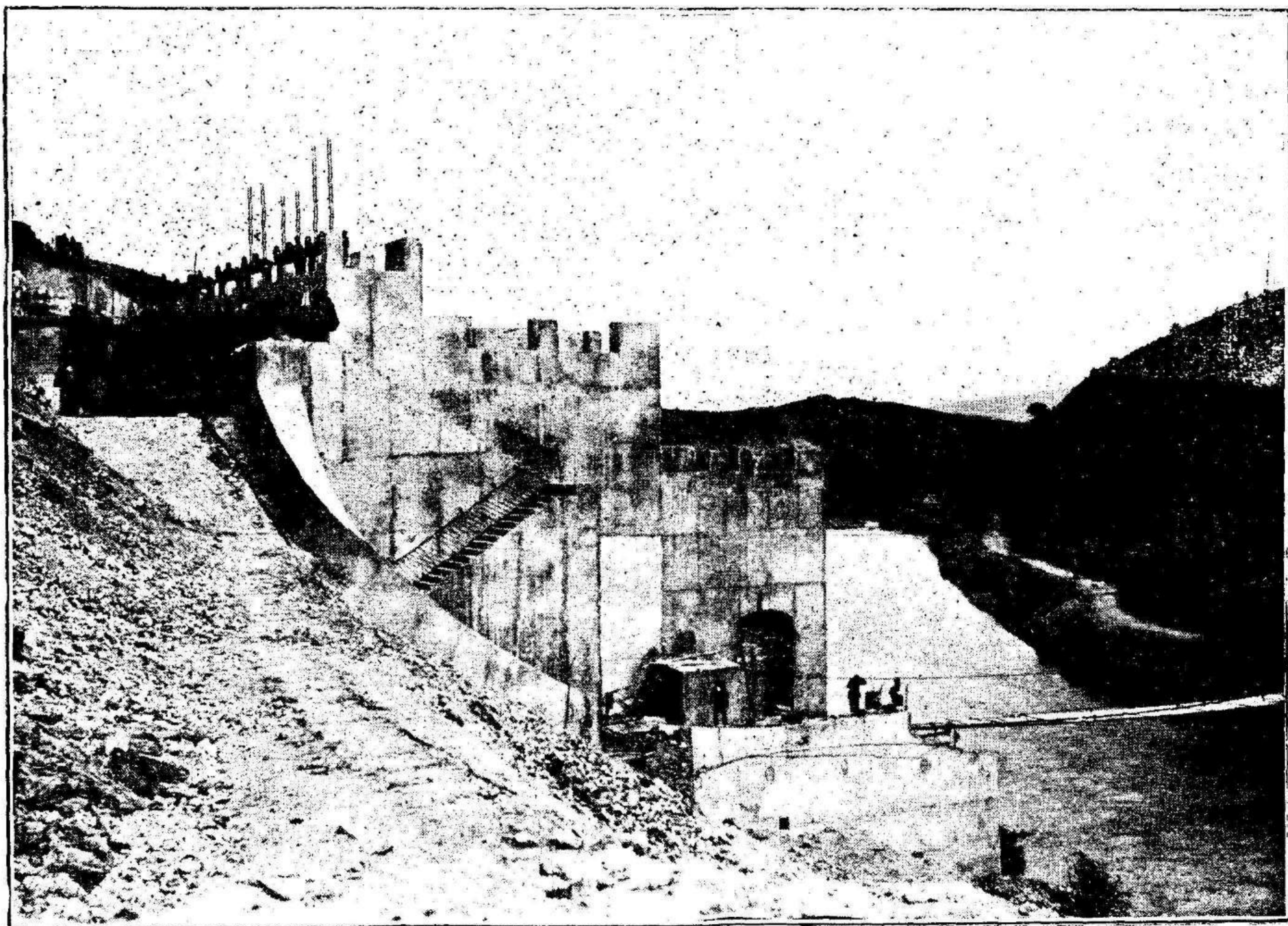
PUENTE DE MANIOBRAS Y ALIVIADERO DE SUPERFICIE
