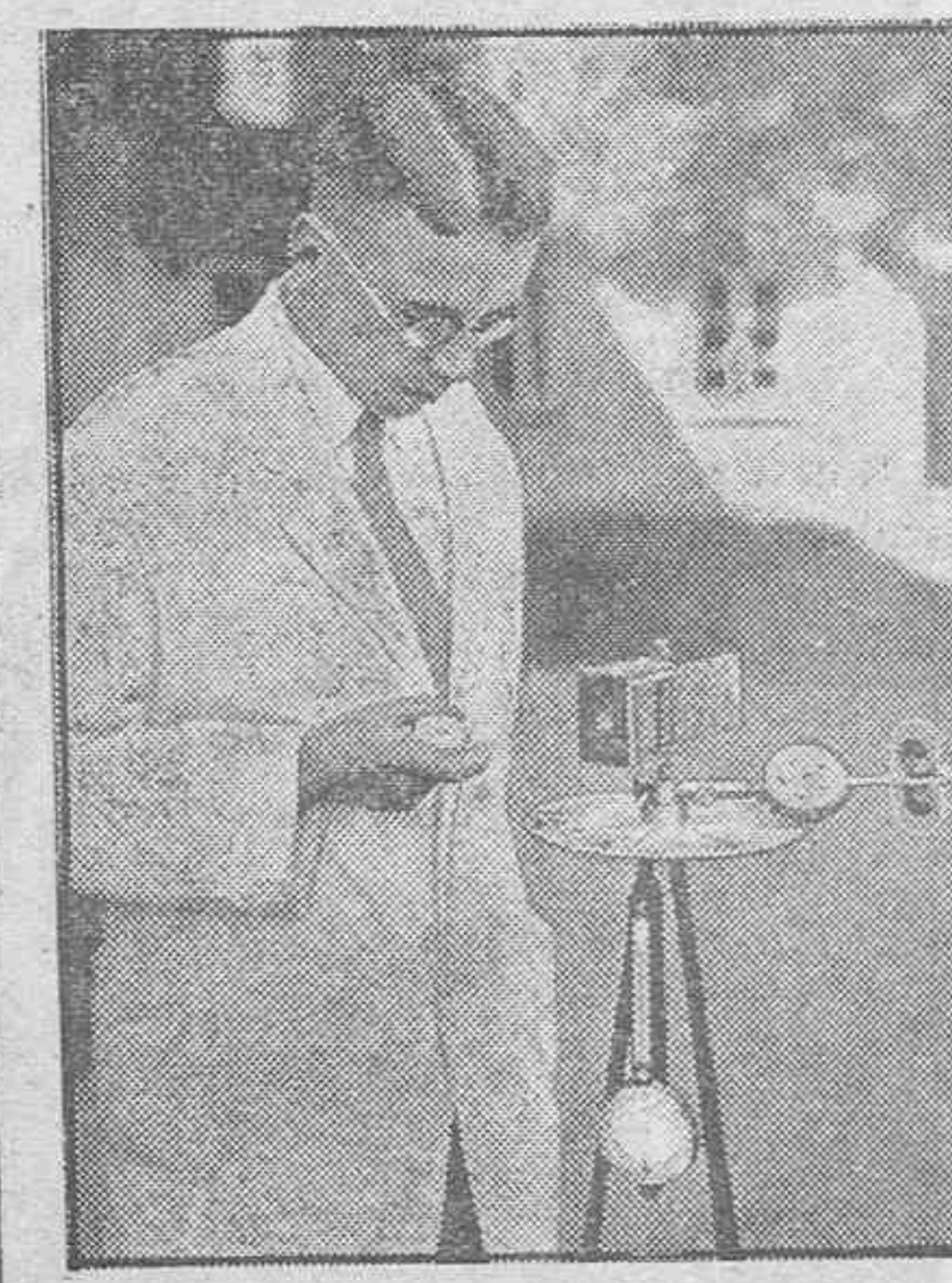
Ingenioso aparato construido en el Instituto prusiano de estudios de higiene, para eliminar las substancias nocivas existentes en el aire.
