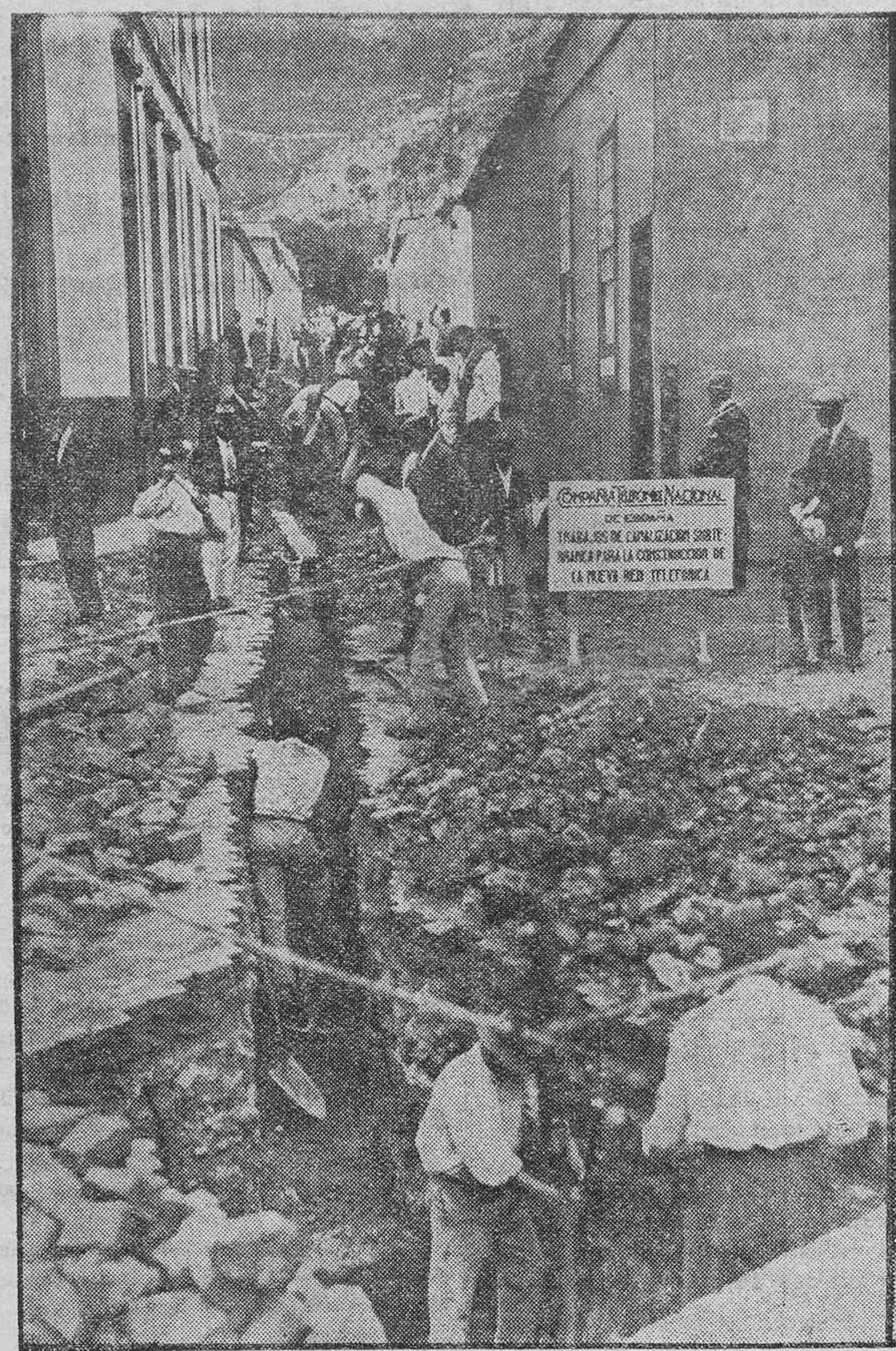
LAS OBRAS DEL TELEFONO URBANO. —Un detalle de los trabajos de canalización subterránea de la nueva red, que viene efectuando en algunas calles de la población la Compañía Telefónica Nacional.—(Foto Benítez.)
