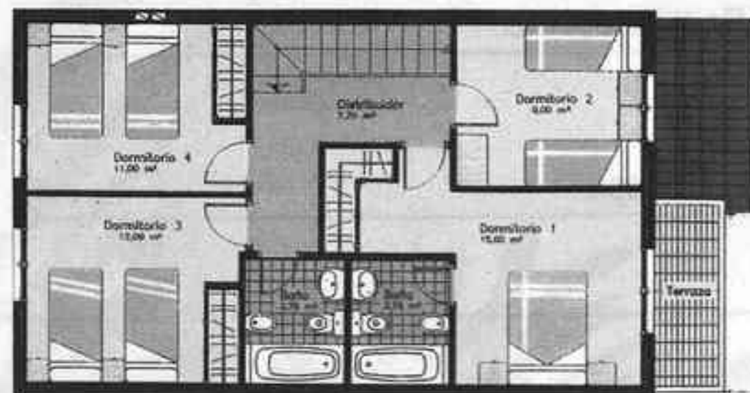
Planta PRIMERA
