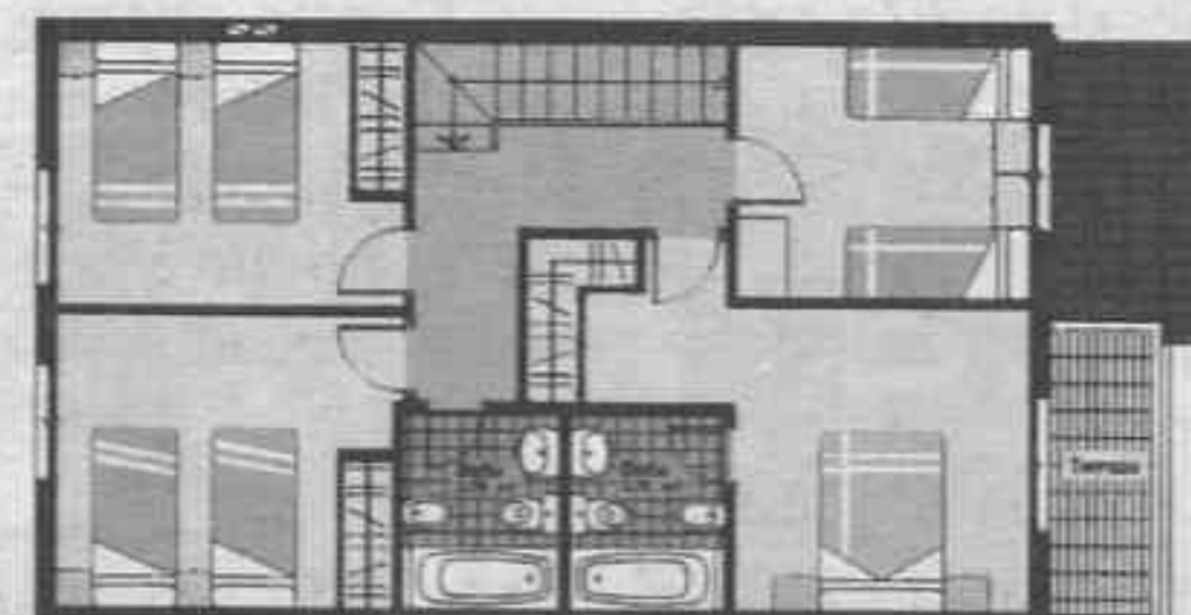
Planta PRIMERA
