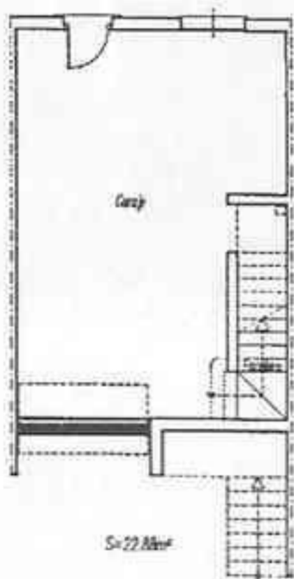
Semisótano (Garaje)
