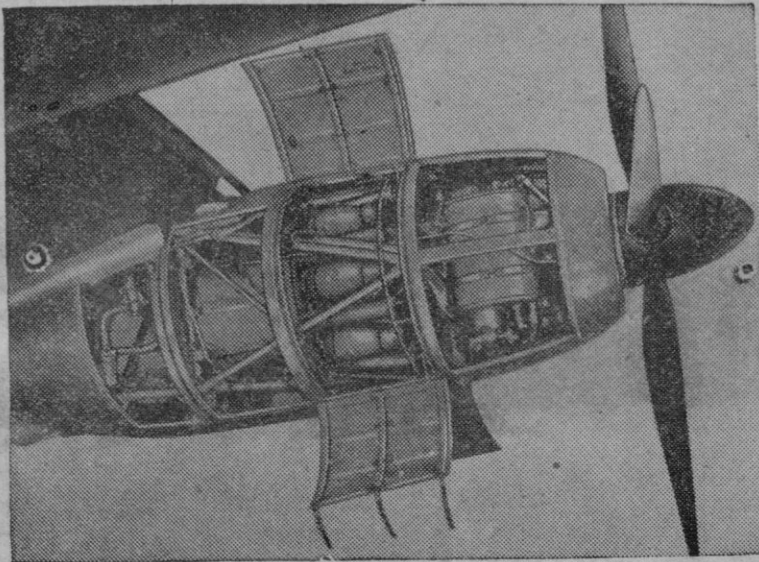
Gran Bretaña a la cabeza en motores a reacción. — El "Theseus", primer turbomotor para propulsión de hélices que se someterá a pruebas oficiales, producto de la Bristol Aeroplane Co. El generador de fuerza de este motor está constituido por un turbomotor de dos pasos que mueve el conjunto combinado de compresor de aire axial y centrífugo, mientras que la hélice está propulsada a través de un tren de reducción, mientras que la hélice está propulsada a través de un tren de reducción epiciclico por un turbomotor separado que funciona como tercer paso antes de propulsar los gases de escape por el tubo de salida. El "Theseus" emplea menos combustible que los motores de reacción actuales
