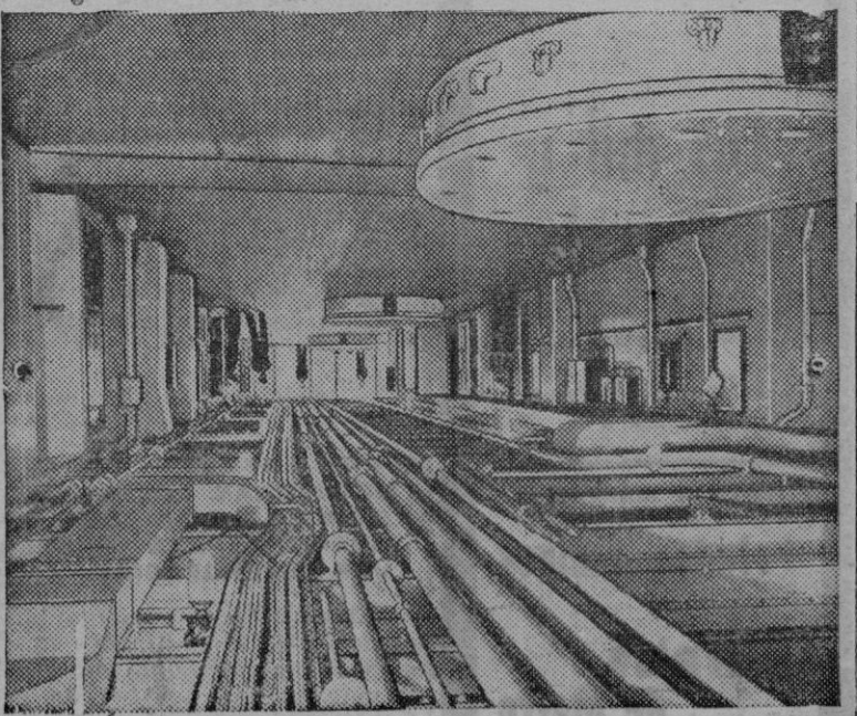
Departamento central del "Monarch", donde se almacenan las grandes bobinas de cable a tender en sus viajes
