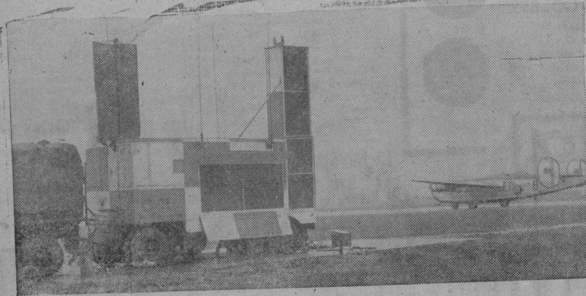
El "radar" aplicado a la Aviación Civil. — Un aparato "Liberator" emprende el vuelo provisto ya de los aparatos de control apropiados. En primer término, la estación del aeródromo instalada sobre un camión de remolque
