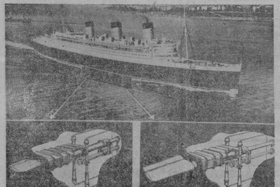
En esta composición fotográfica, vemos, por debajo de la línea de flotación, los estabilizadores del trasatlántico inglés «Queen Mary», con el detalle de dichos aparatos, que son utilizados para compensar los movimientos del buque cuando hay mala mar.
