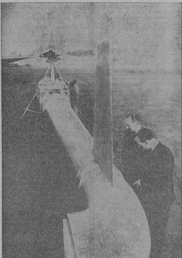
En una Exposición aérea que se celebra en Radlett (Inglaterra), figura este extraño helicóptero a propulsión por cohete fabricado por la empresa Gunlitte Owen. Funciona con un sistema de control torque y tiene un motor Gipsy VI Serie IX de la Casa De Havilland
