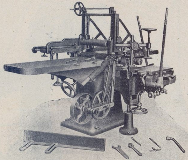
MODELO TF MÁQUINA "UNIVERSAL"
