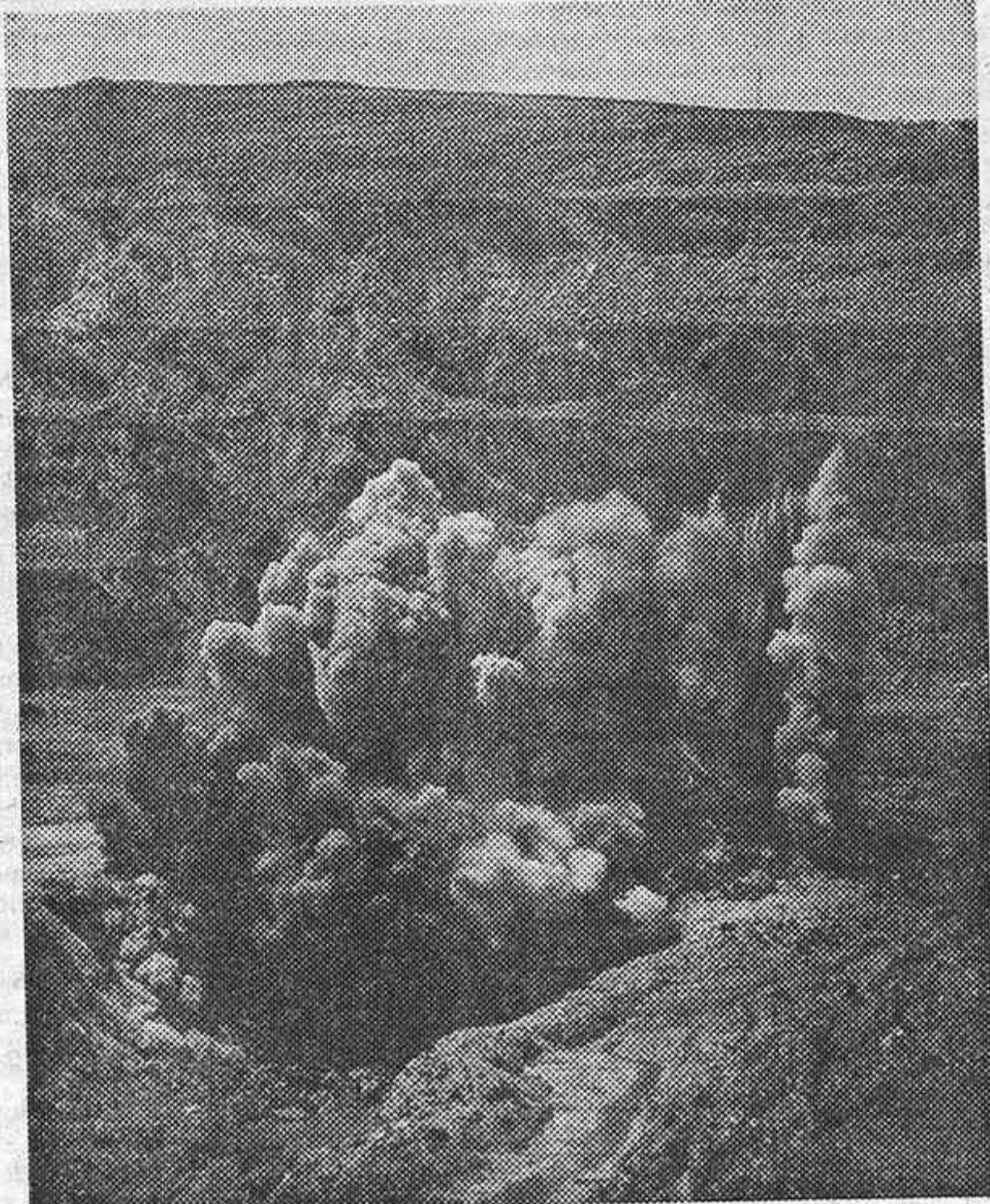
Detalle de una voladura en la corta de la mina
