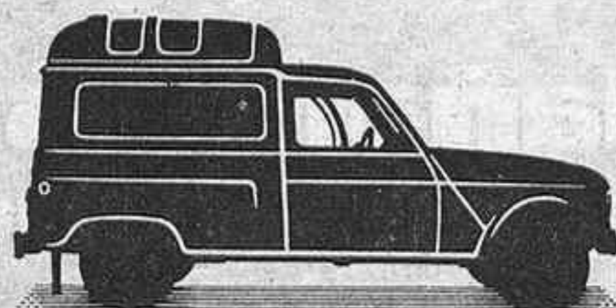
Sobreelevada Carga 425 kg. Altura útil 1,307 m. Volumen útil de carga 2.08 m³
