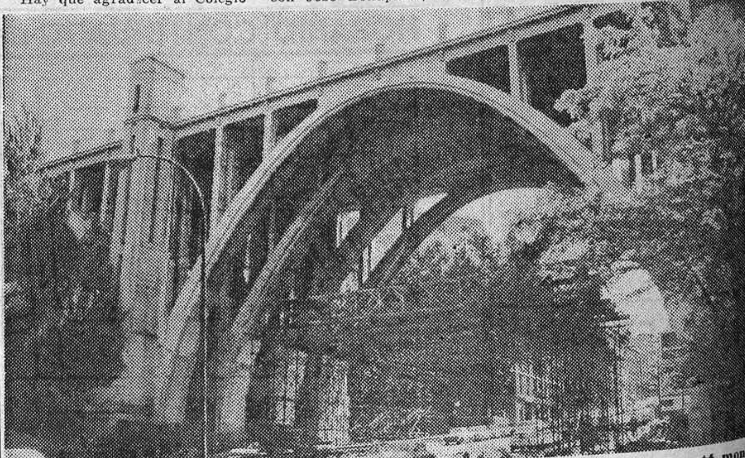
Del Viaducto, que persistirá como hasta aquí, va a repararse únicamente la calzada. Ya está montado el necesario andamiaje, que se advierte aquí bajo el arco central. A la izquierda, la torreta de uno de los dos ascensores que unirán en vertical las calles de Segovia y de Bailén. (Torremocha.)
