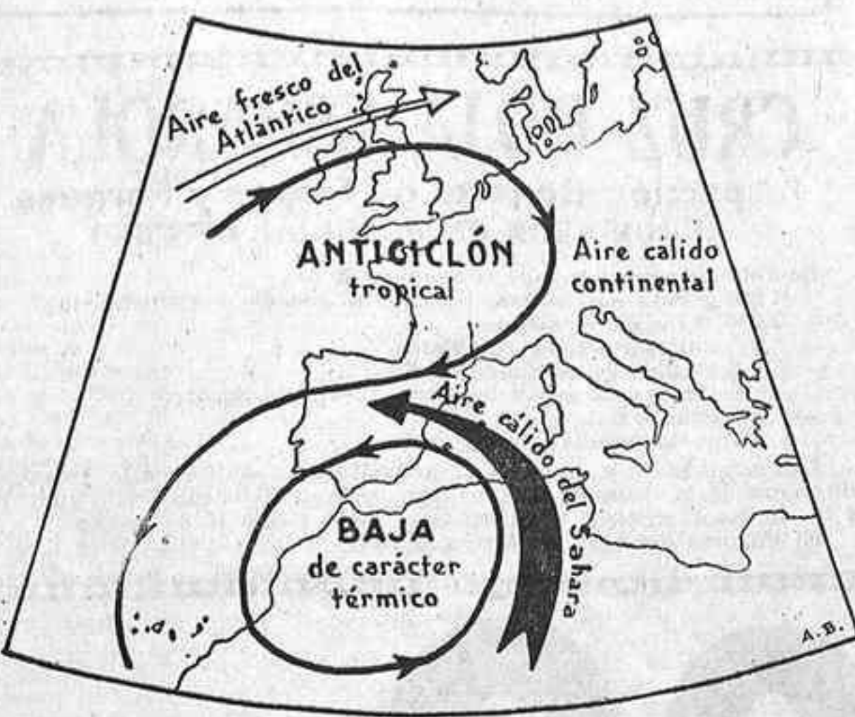
Esquema representativo de una "ola de calor". Penetración en España de aire cálido y seco del Sahara y del continente europeo. (Dibujo del autor.)
