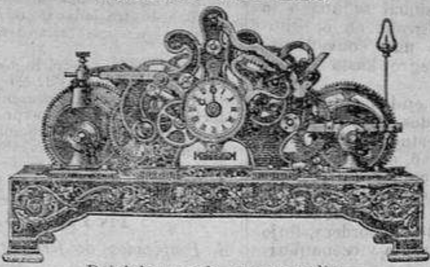
Reloj de torre de oras y meias
