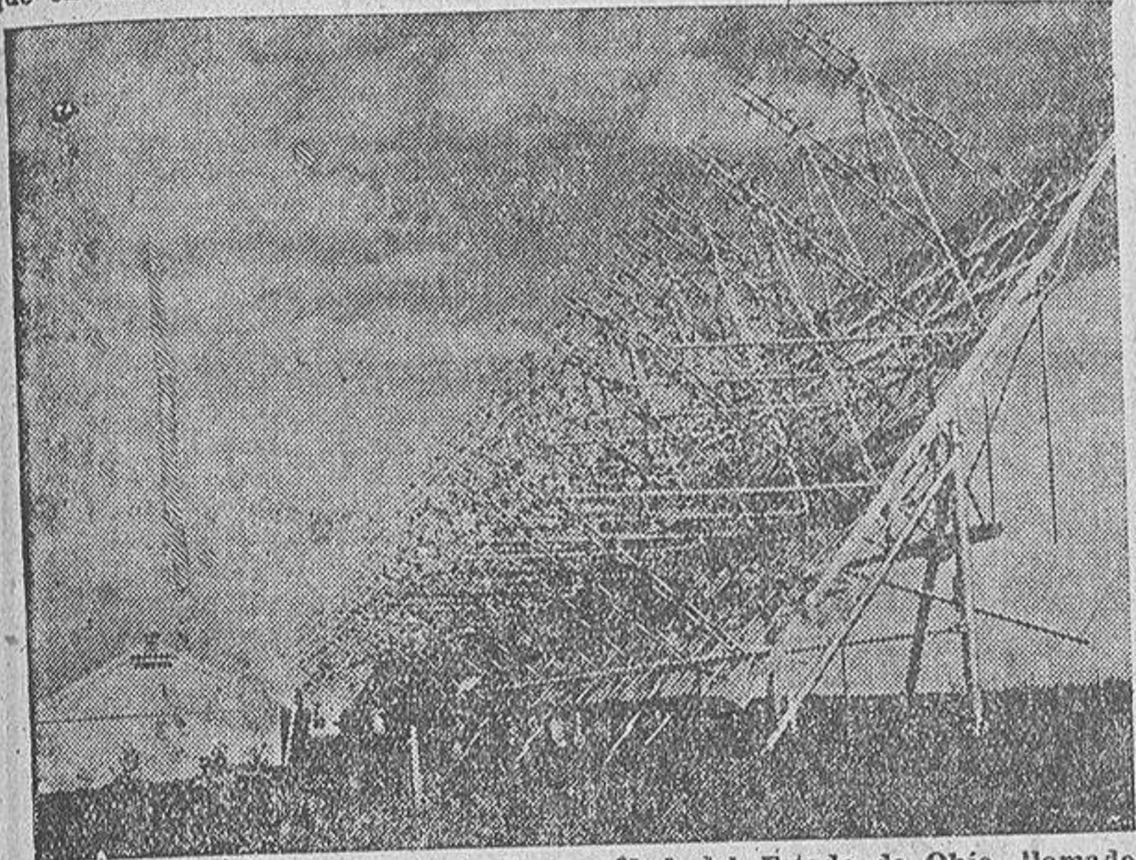
Este es el radiotelescopio de la Universidad del Estado de Ohio, llamado jocosamente "el colchón de muelles", por sus 96 antenas en espiral. Desde su construcción, en 1952, los astrónomos norteamericanos han escuchado las radiosondas procedentes de Júpiter, Venus y Marte, planeta este último cuyas condiciones de vida preocupan especialmente a los científicos de los espacios siderales
