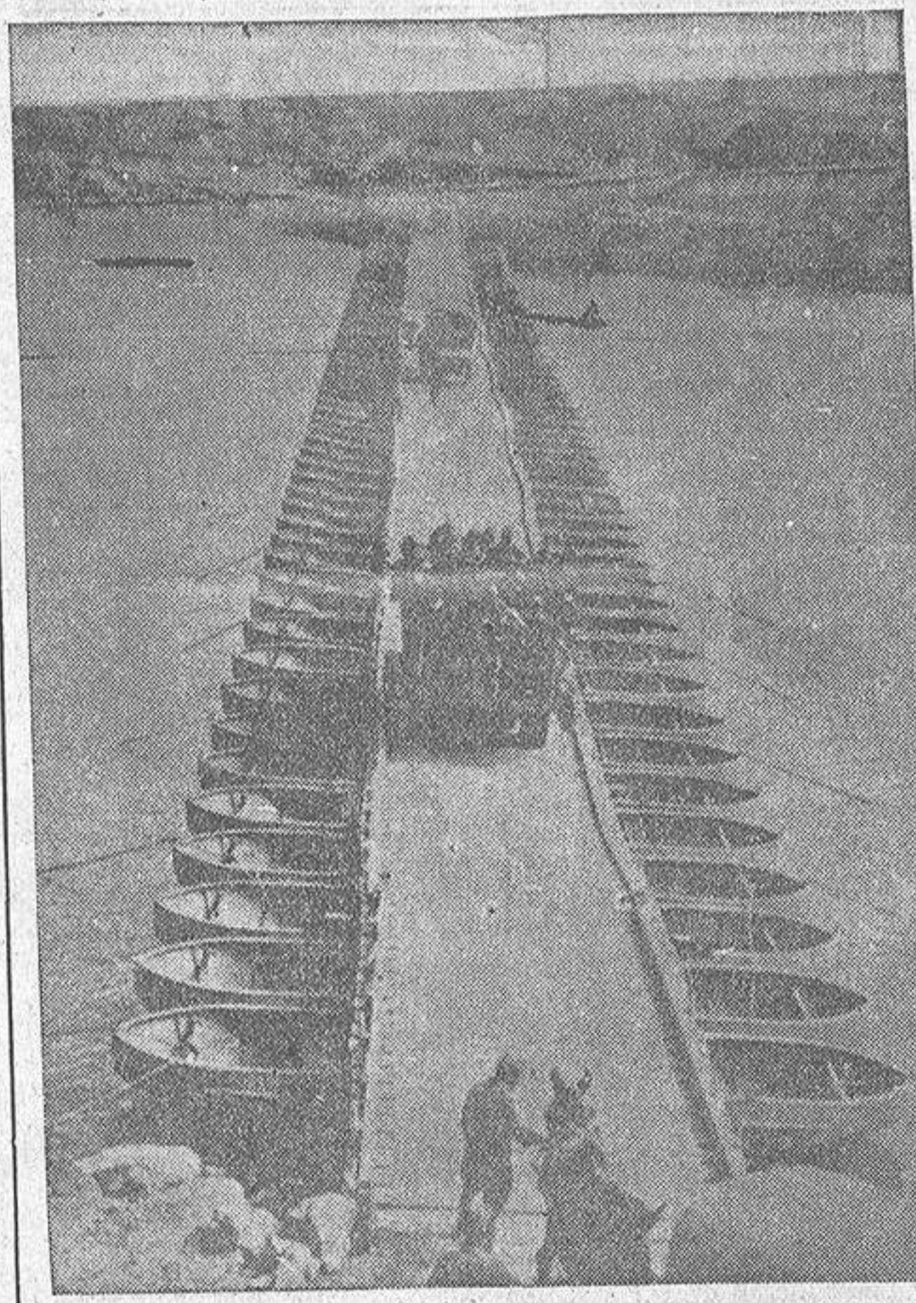
Para atravesar el río Cinca, cuyos puentes volaron los rojos con el intento inútil de bloquear el avance de los nacionales, los ingenieros del General Franco construyeron inmediatamente este magnífico puente de barcas sobre el que pasaron las fuerzas que, rápidamente, conquistaron la población de Fraga, y días después, la ciudad de Lérida
