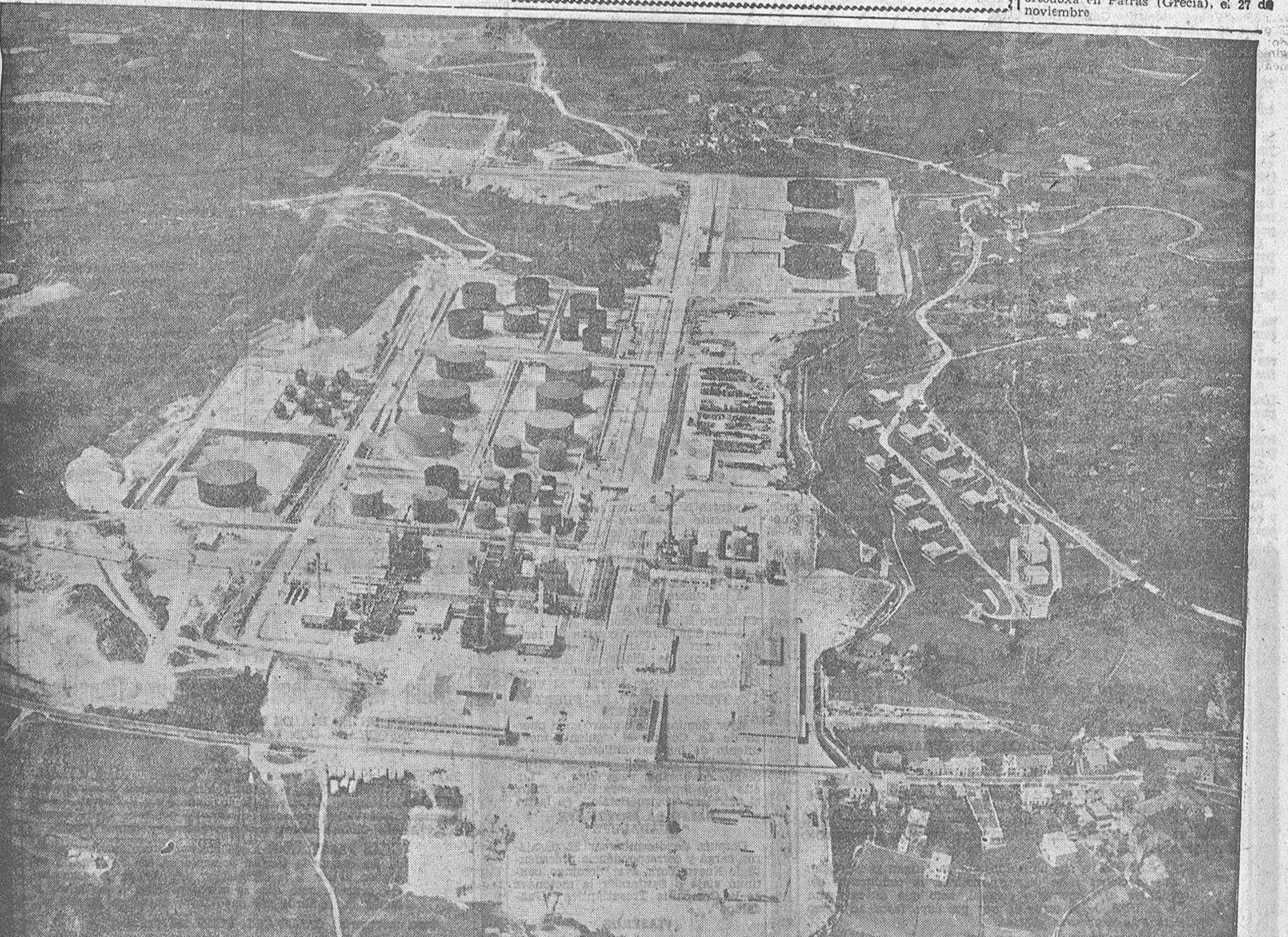
Vista aérea de la Refinería del Noroeste de España de la Compañía Ibérica Refinadora de Petróleos, S. A. "Petroliber" cuyas pruebas se realizan a un ritmo y resultado plenamente satisfactorios.
