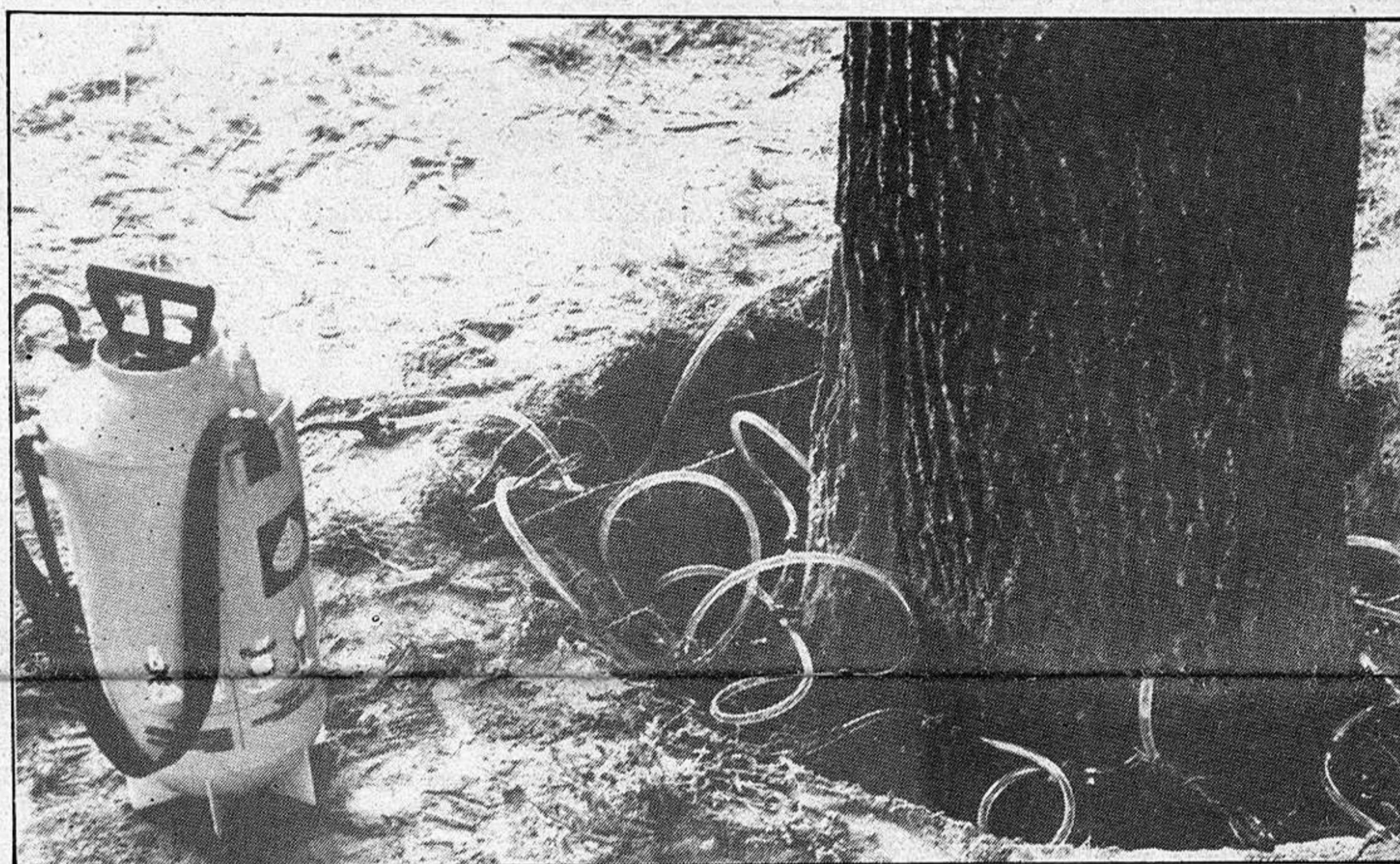
En la imagen se puede apreciar el depósito del líquido protector y la aplicación de las boquillas en la base del tronco del olmo (Foto: J.A. Guardiola)
