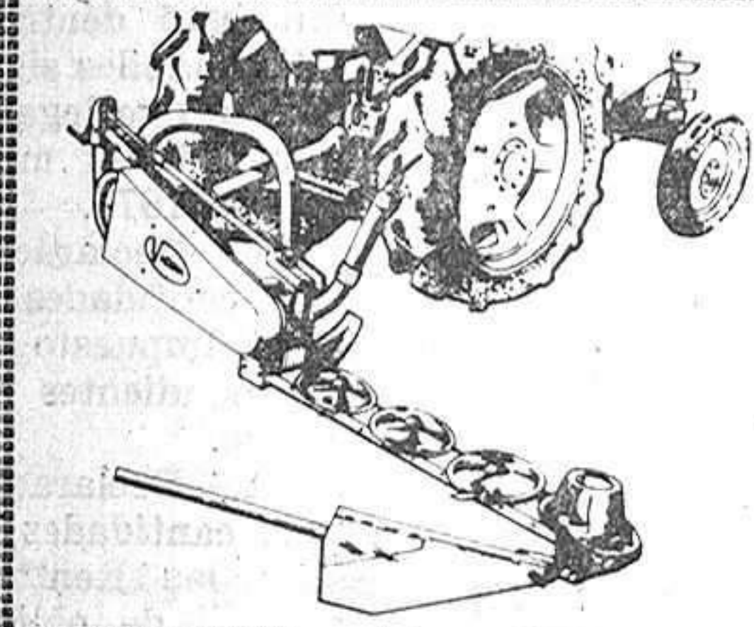
SEGADORA ROTATIVA, con 4 discos a 3.200 r.p.m. corta forraje en un ancho de 1,60 m. a 15 Km. hora
