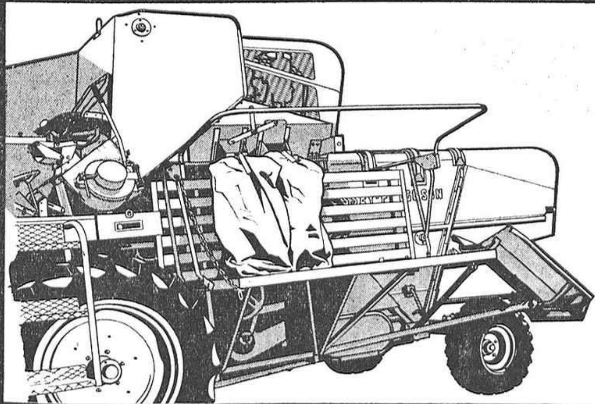
LA MISMA COSECHADORA DISPUESTA PARA TRABAJAR CON ENSACADOR
