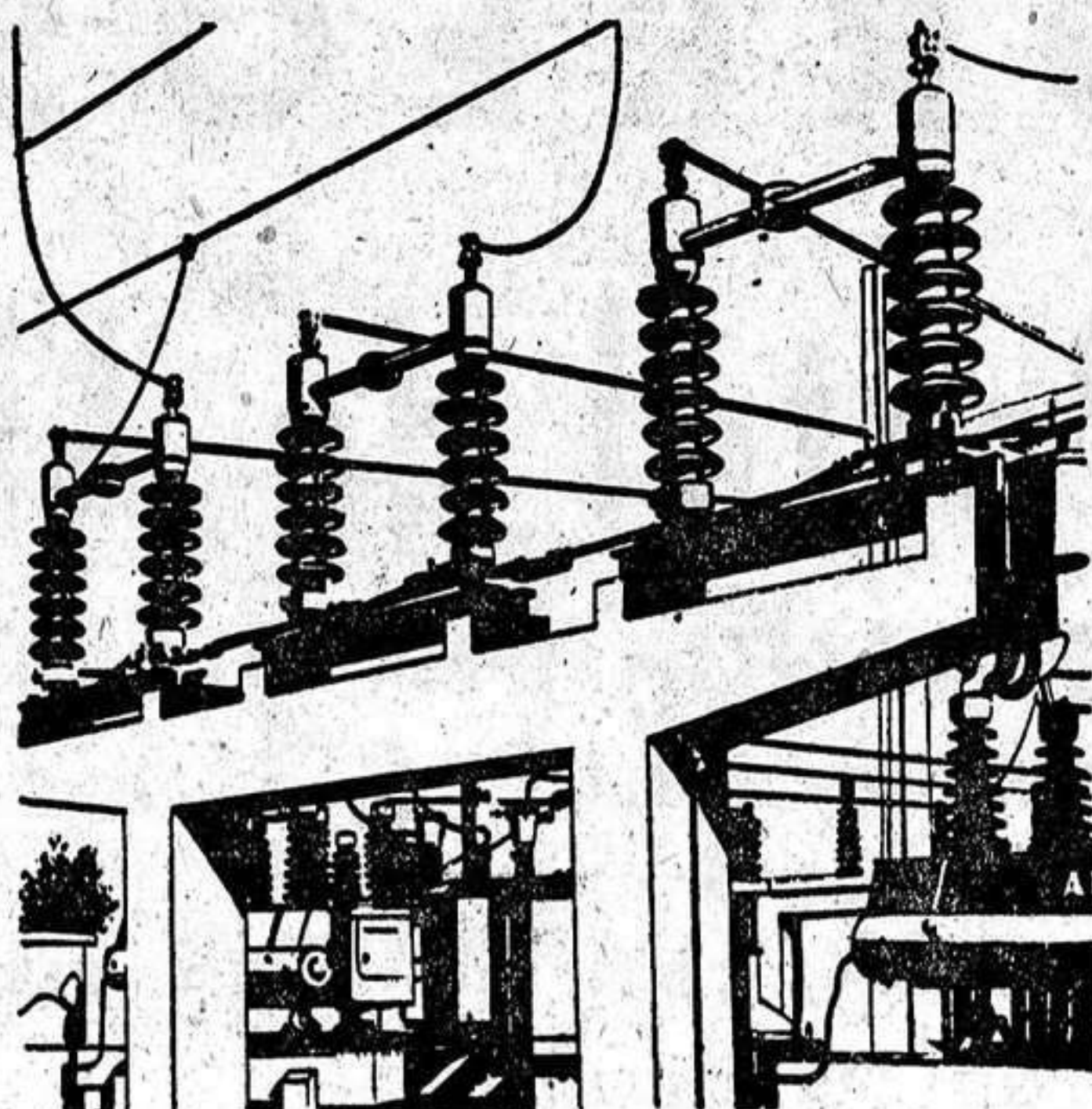
Seccionador tripolar para 66.000 Voltios, 600 Amperios
