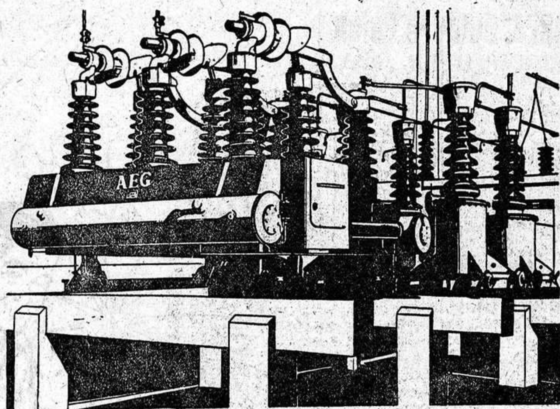
Interruptor de aire comprimido para 66.000 Voltios - 1.000 Amperios, capacidad disruptiva: 1.500.000 KVA.
