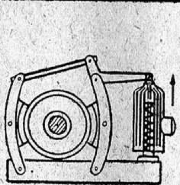
Freno y regulación.
