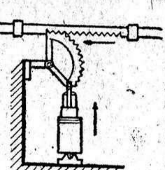
Accionamientos por cremallera.
