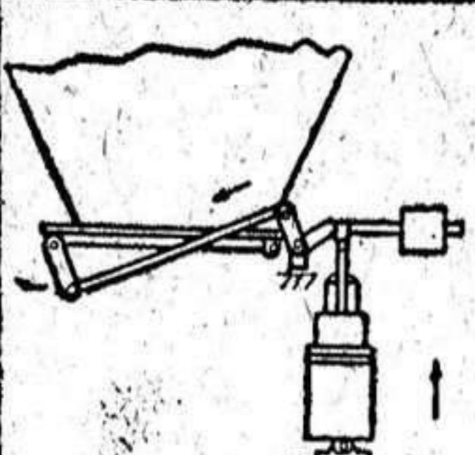
Tolvas y pesaje automático.
