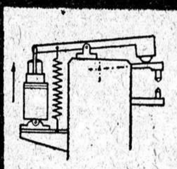
Máquinas de soldar por puntos.
