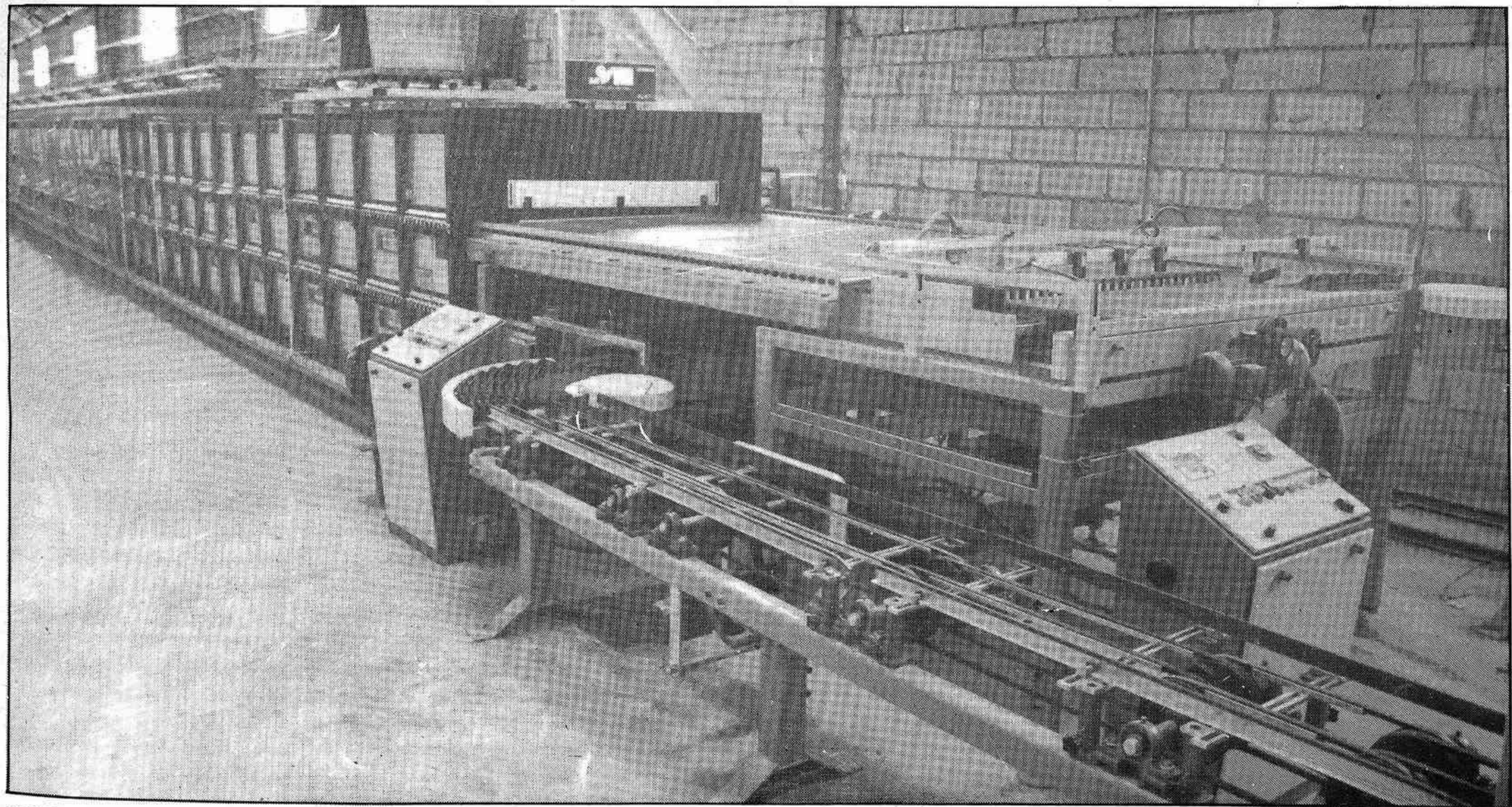
CERAMICA NULENSE, vista interna de la nave con la nueva instalación de monococción rápida. Horno de 56 mts. de longitud de do: canales, hecho por SITI-IBERSITI
