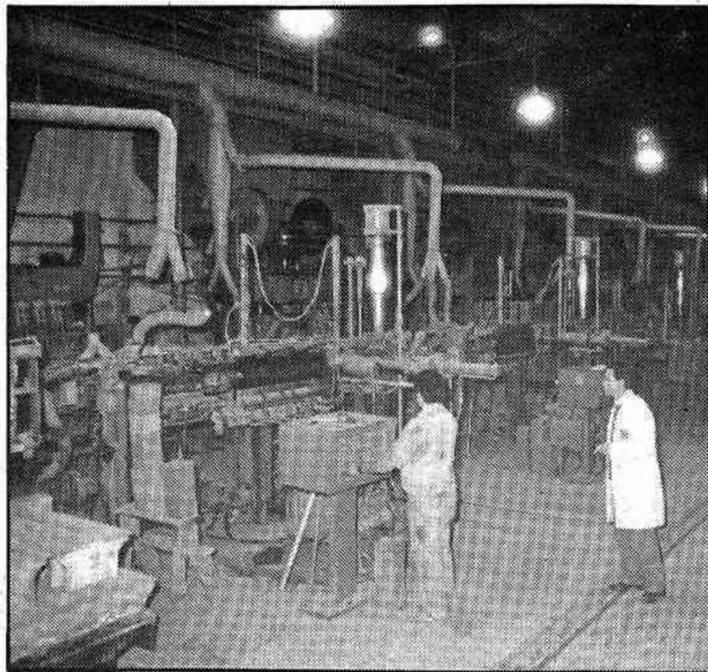
Prensas. Es el segundo paso del proceso
