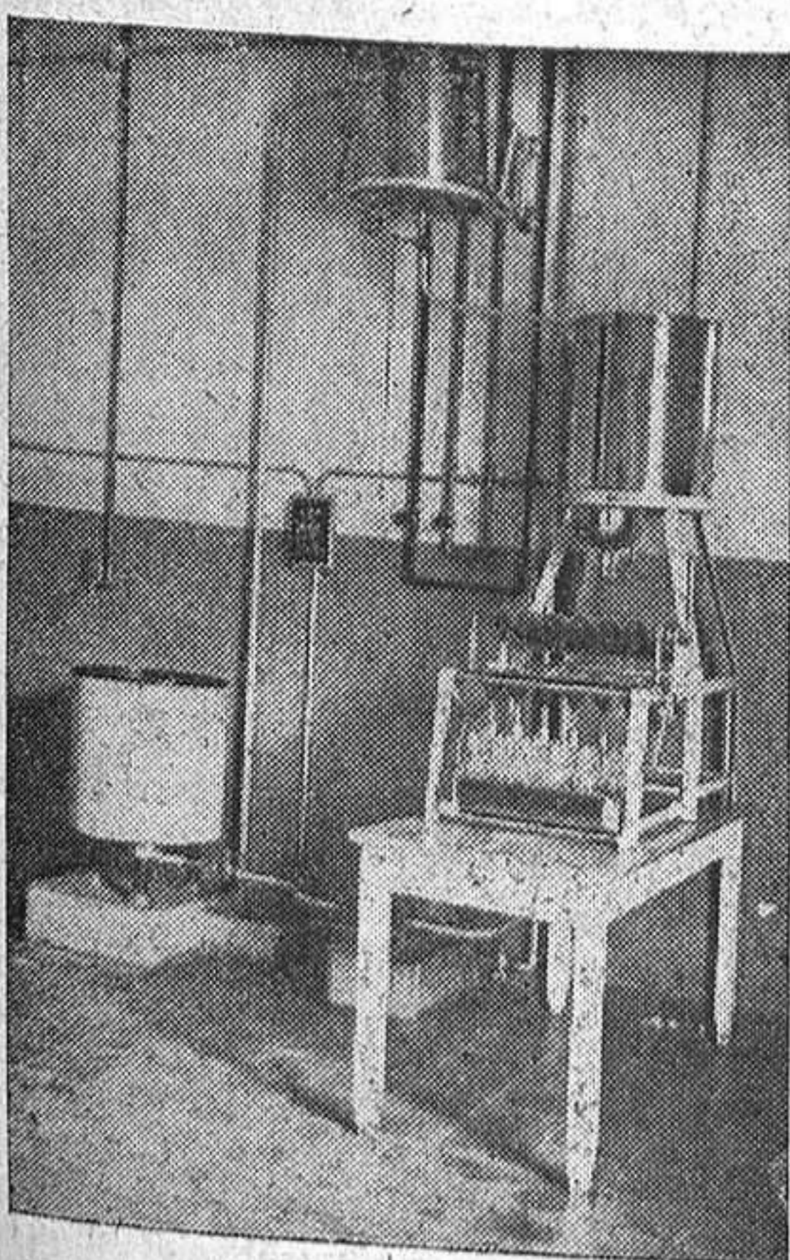
Instalación electro-automática para el envasado y medida de leche que luego se esteriliza.
