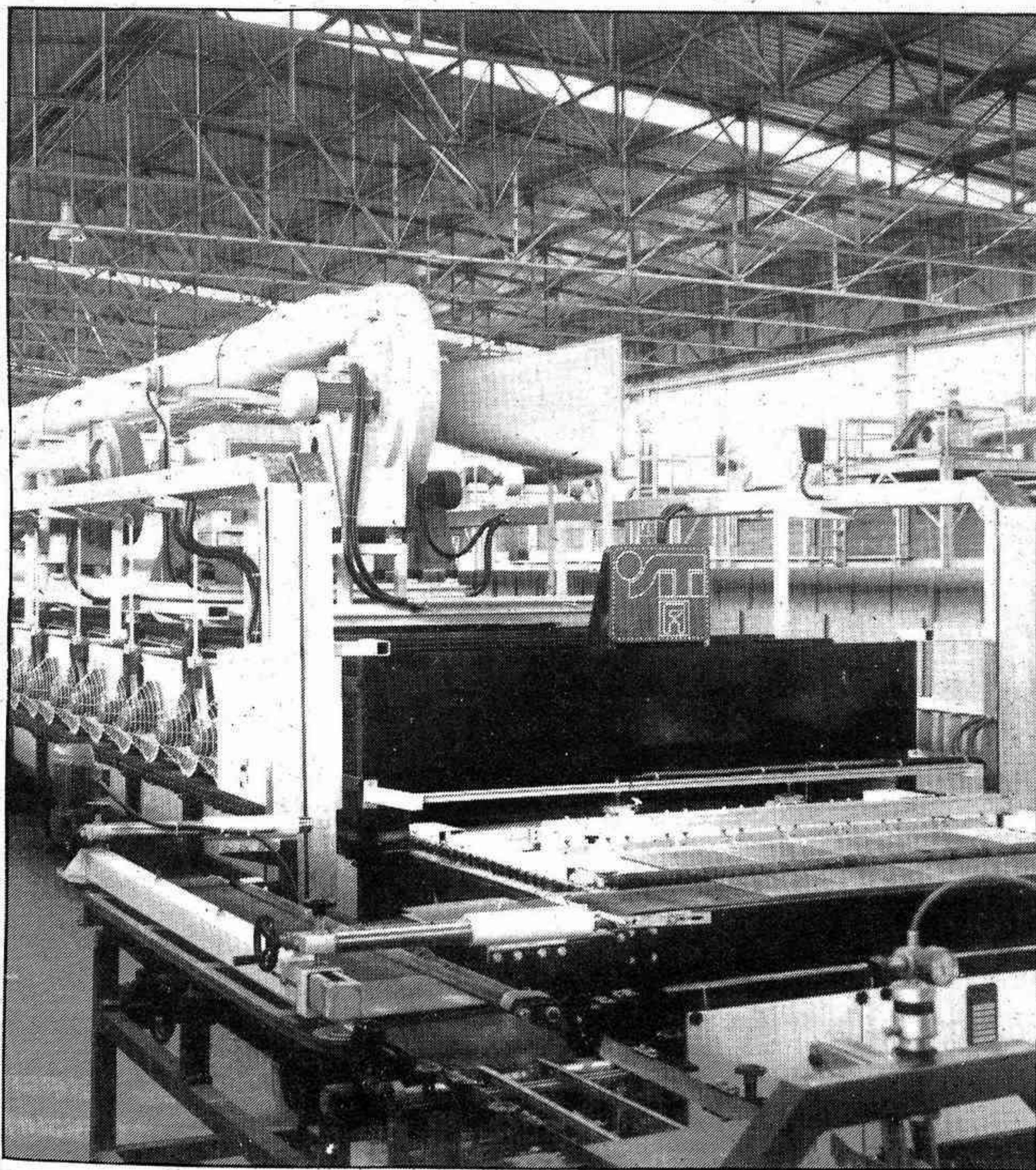
IBERSITI, S. A., Castellón (España) bajo licencia de SITI, S. p. A. Marano Ticino (Italia). Horno tipo FILX de 60 m.
