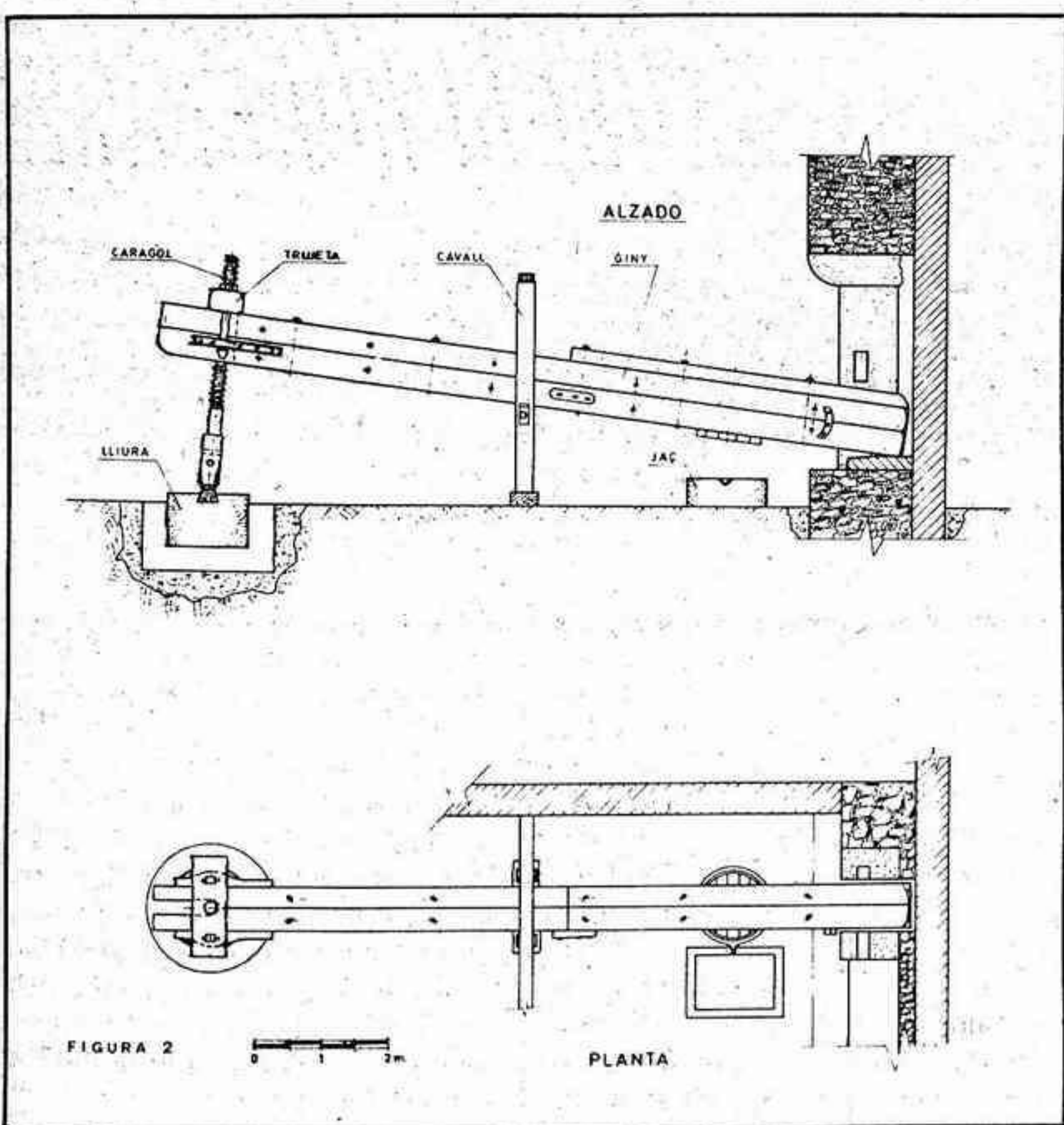
Alzado y planta de la prensa
