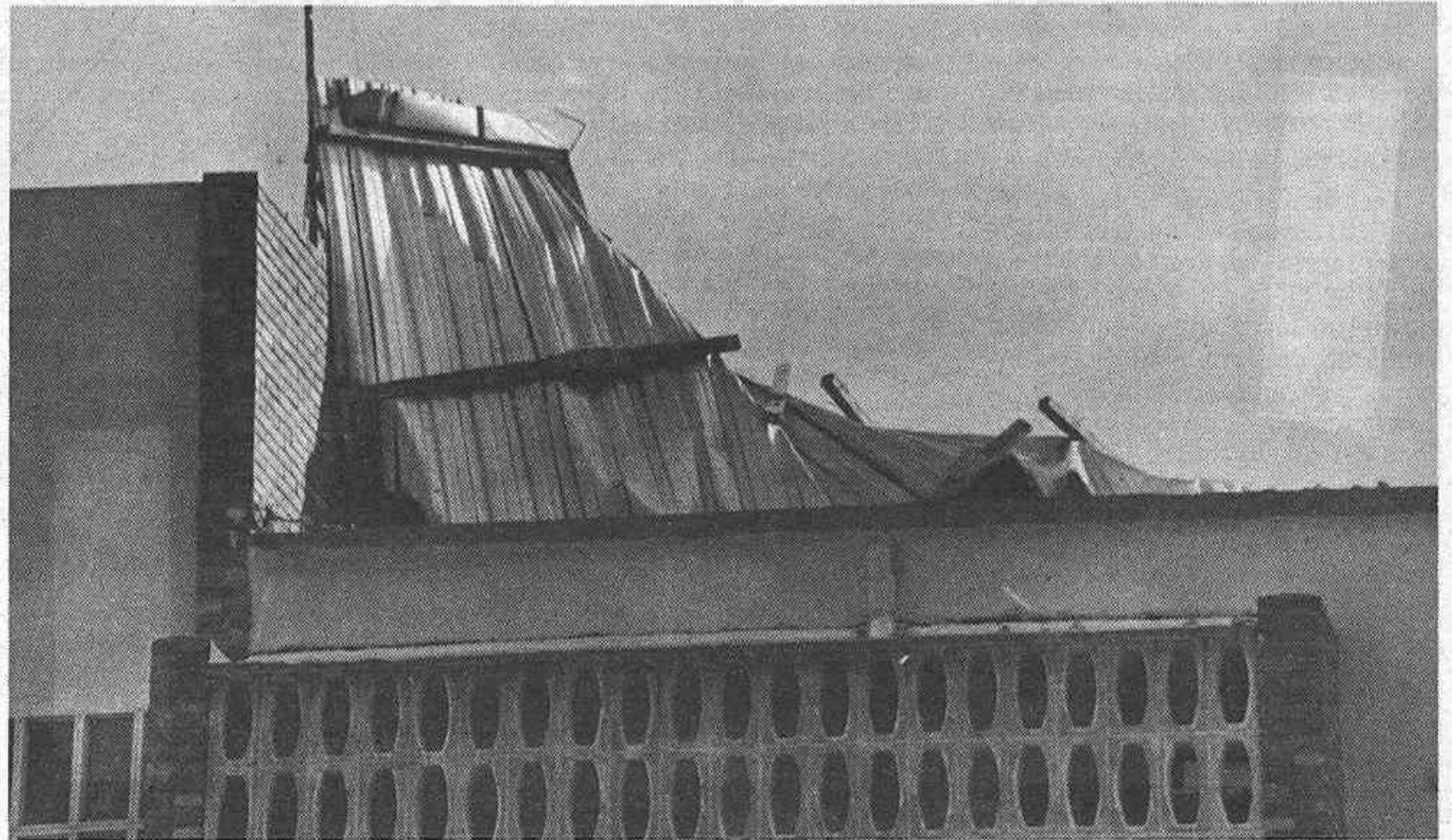
Los restos de la cubierta que quedaron sobre el edificio.
