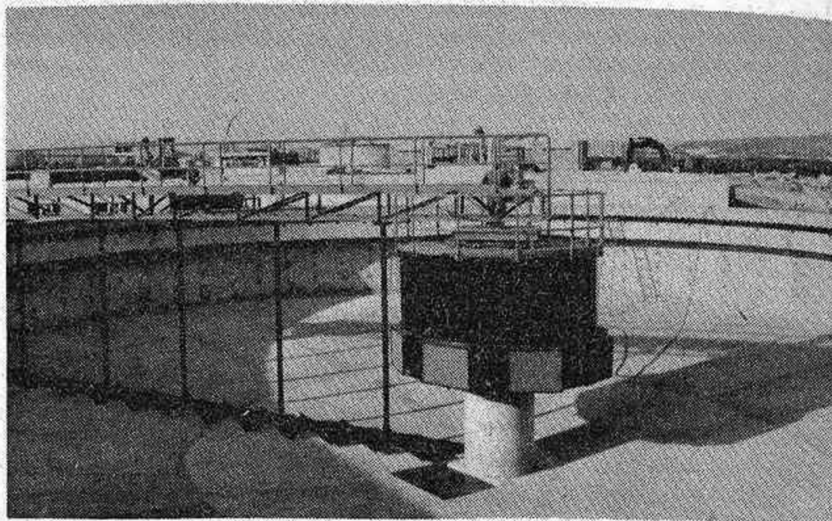
Vista de las instalaciones de la Estación Depuradora.
