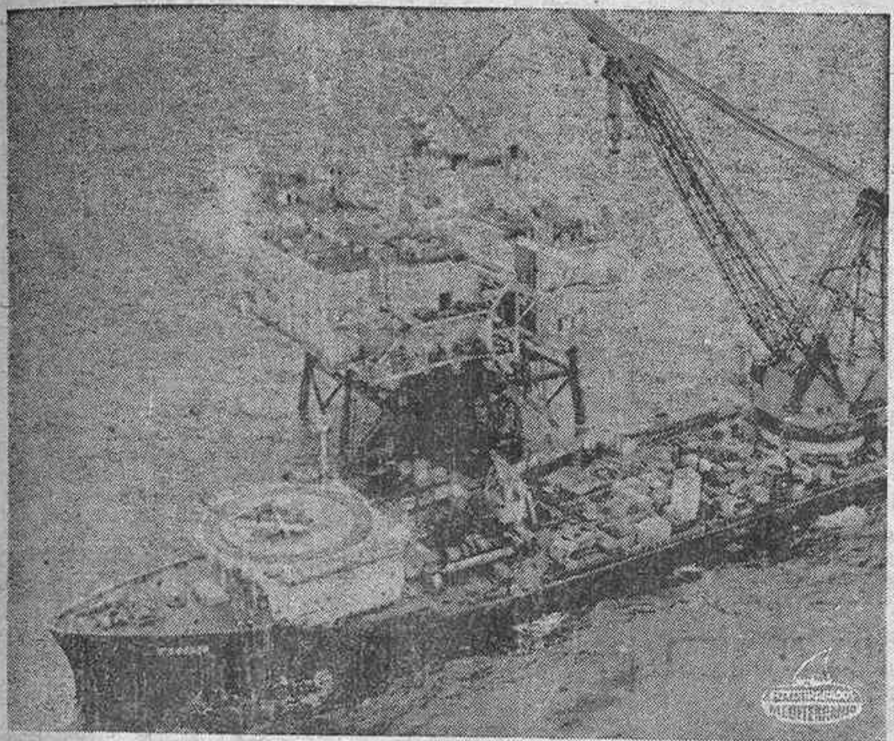
ABERDEEN (Escocia). — La mayor grúa flotante del mundo, a bordo de la barcaza "Thor", después de completarse la instalación de los módulos de 500 toneladas sobre la plataforma de producción petrolífera "Graythorp 1" de la BP, en el yacimiento petrolífero "Forties" a 110 millas de Aberdeen. La instalación fue demorada tres meses a causa del mal tiempo reñanante, suponiendo los gastos 240.000 dólares diarios. La perforación se iniciará en la primavera próxima. — (Telefoto Cifra Gráfica-Upi)
