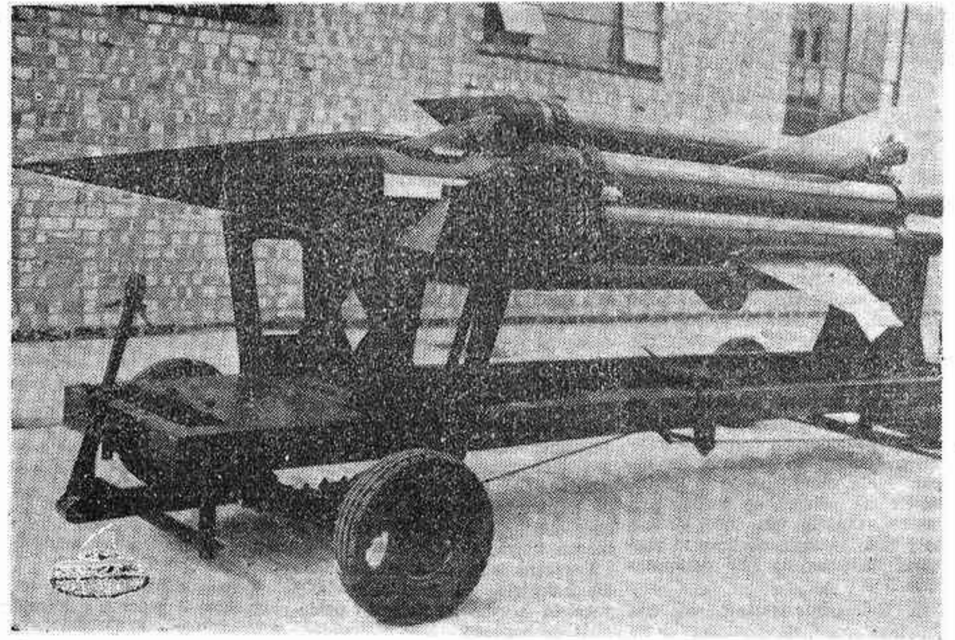
Proyectil dirigido, construido por la casa aeronáutica inglesa «Armstrong»
