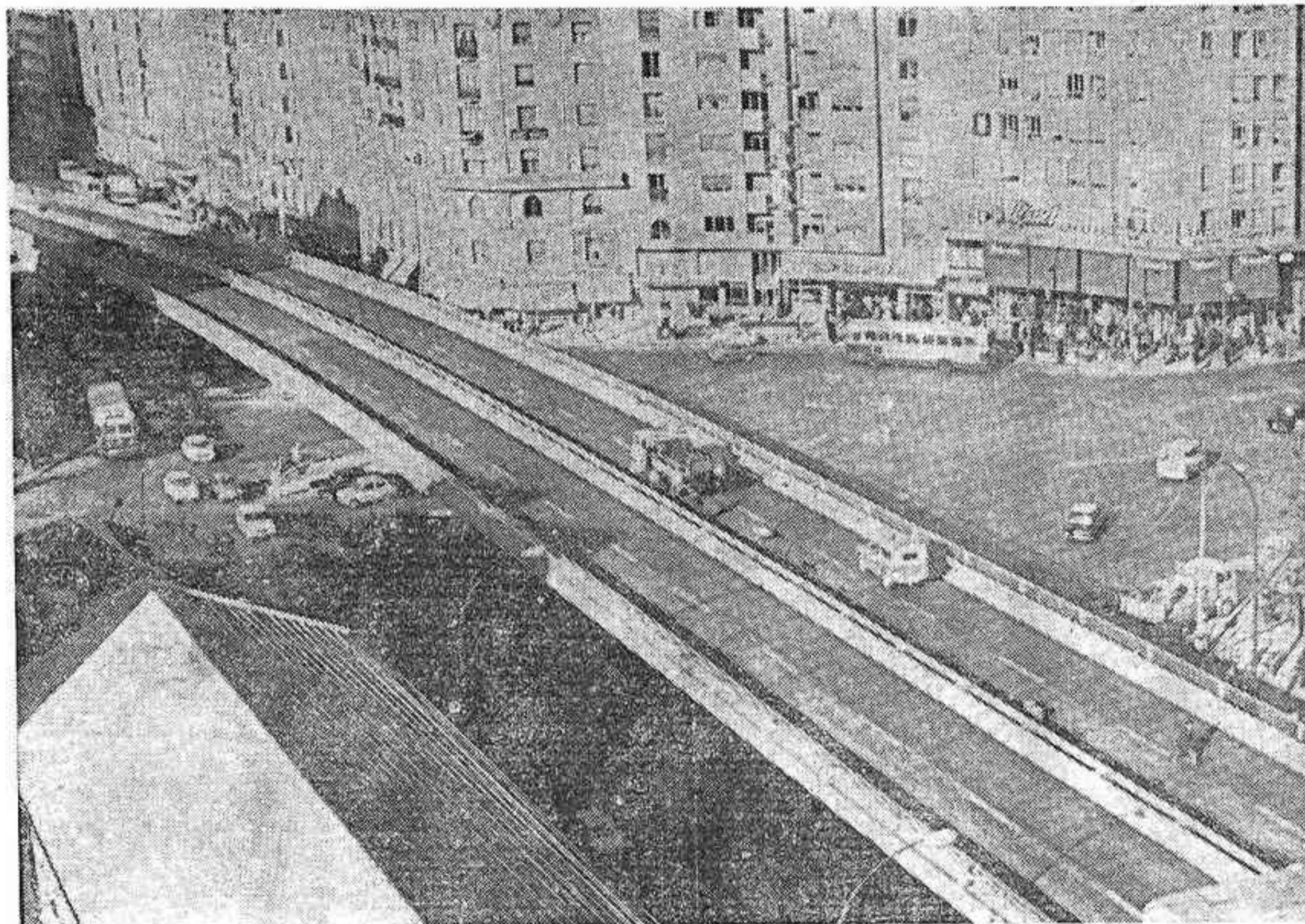
MADRID. — Este es el paso elevado que se ha construido en Cuatro Caminos. Contribuirá de una manera extraordinaria a resolver el problema del tráfico rodado que existe en aquella zona madrileña. Su inauguración es inminente. A manera de prueba, se le ha hecho soportar un peso de 480 toneladas. — (Foto CIFRA)
