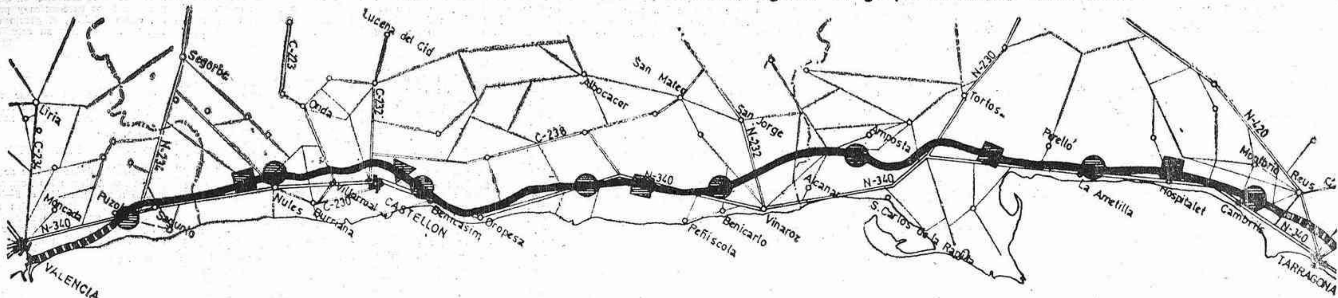
Plano de situación, a escala 1:400.000, del tramo de autopista Tarragona-Valencia. El trazado discontinuo representa los tramos sin peaje; el trazado negro grueso es la autopista en sí y las restantes vías señaladas, las carreteras estatales. Los círculos rayados representan la situación de las áreas de servicio; los cuadrados, las áreas de mantenimiento; el triángulo, la zona de servicio especial.
