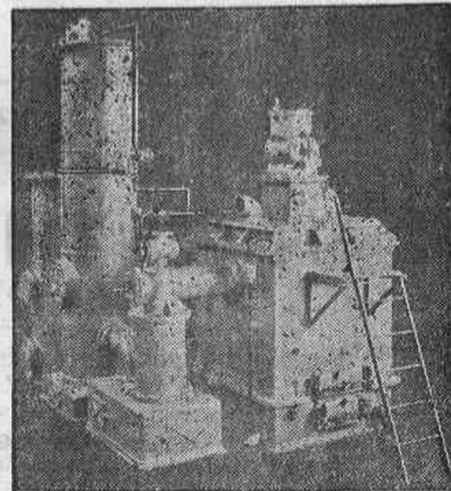
Gasógeno sencillo
