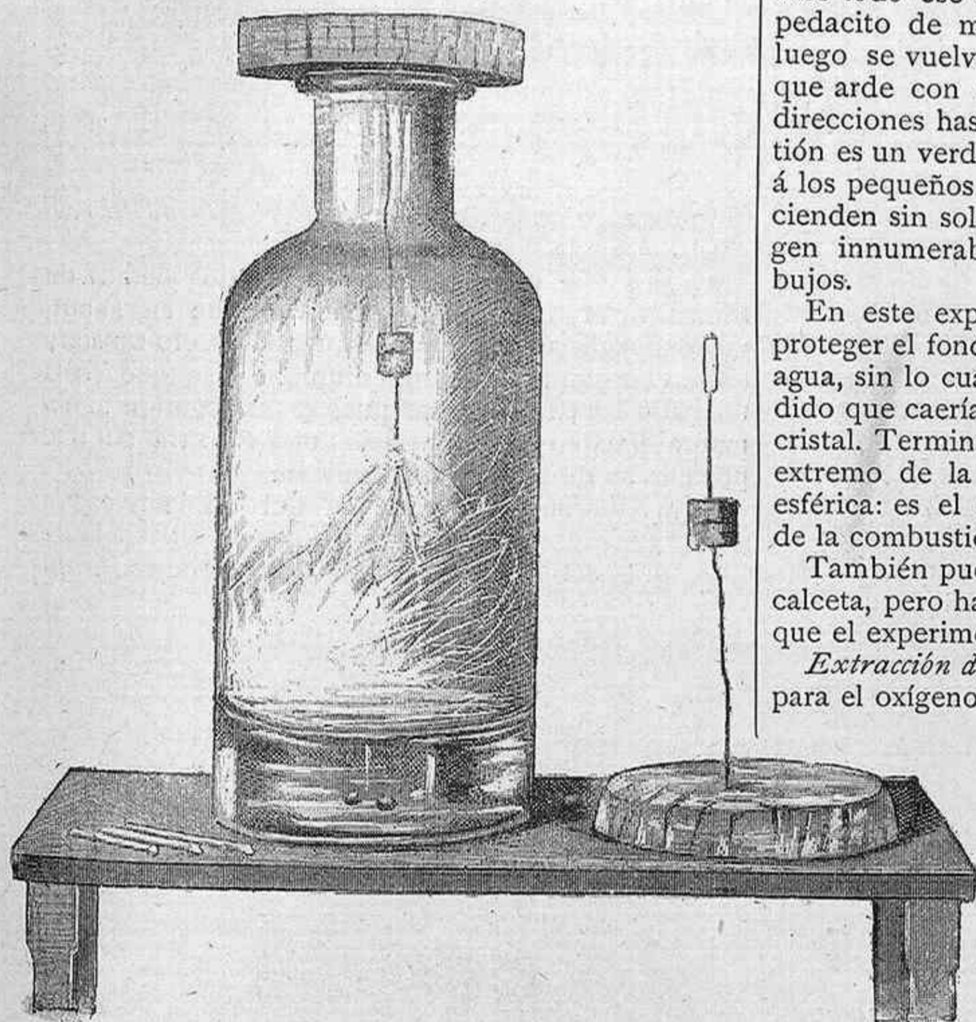
EL OXIGENO. - Fig. 2. Combustión en el oxígeno de una aguja de coser
