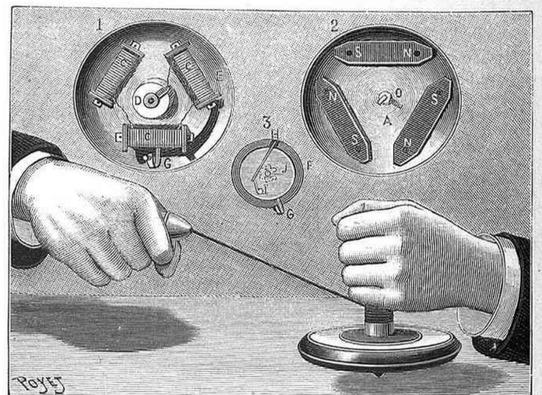
Trompo electro-magnético. - Modo de hacerlo funcionar y detalle del mecanismo
