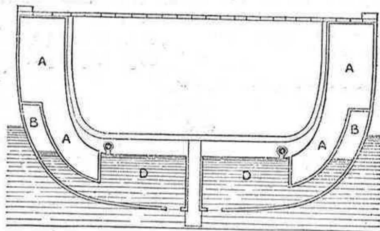
Fig. 3. Sección transversal del barco insumergible DD Water-ballast. - A, A, A, A, B, B, cajones de aire comprimido.
