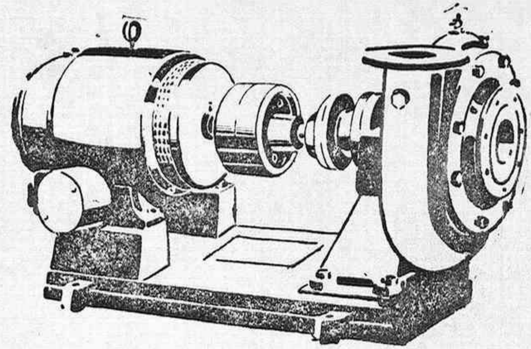
Grupo electro-bomba de baja presión
