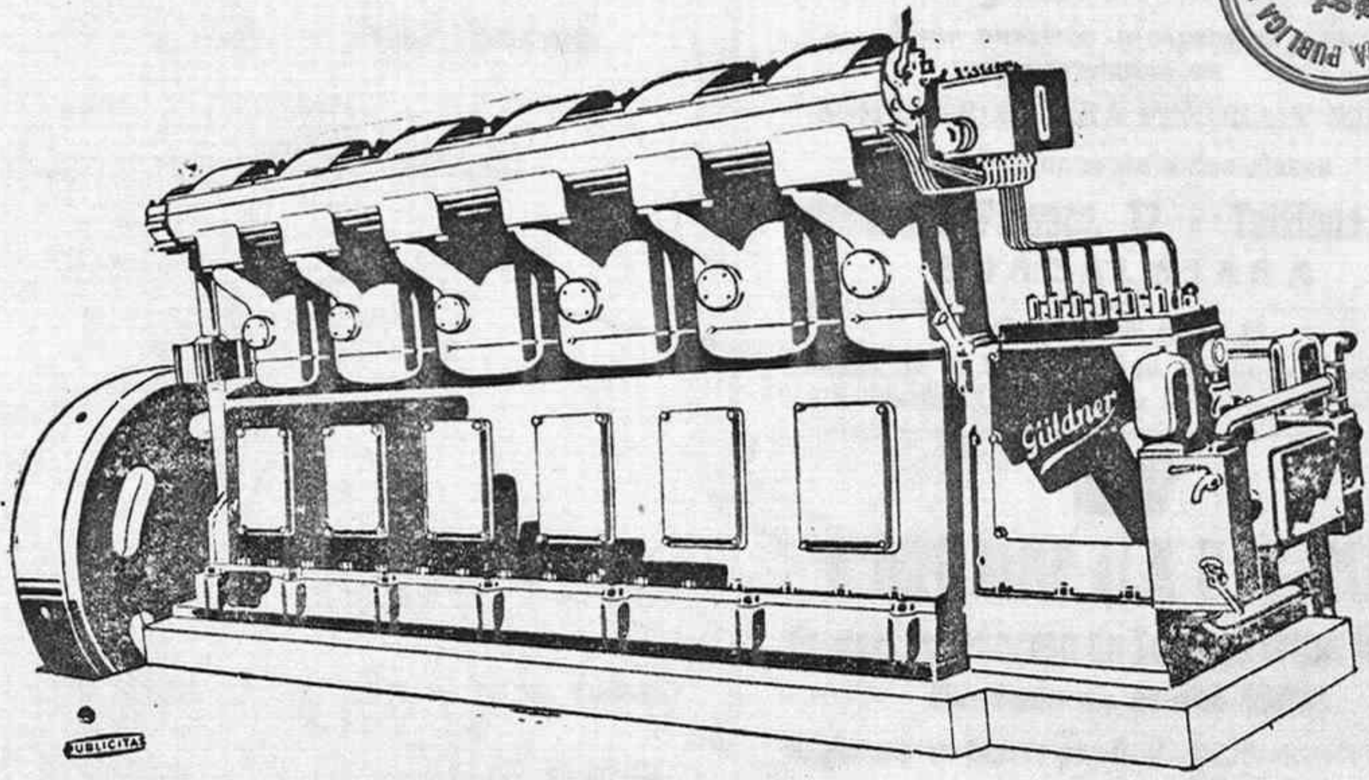
Motores Diesel «Güldner» hasta 1.200 caballos
