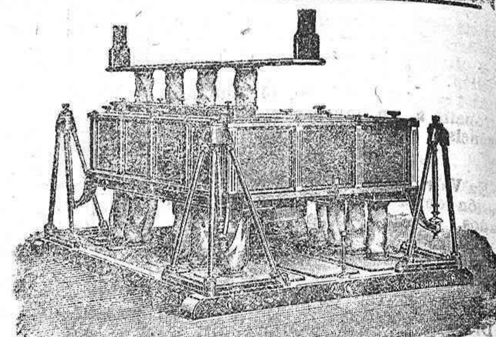
Plansichter DAVERIO construcción, 1902
