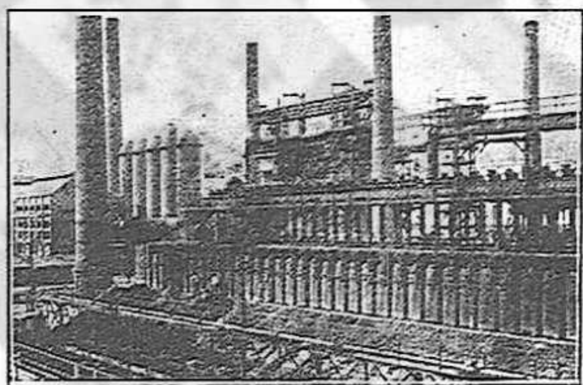
Quaranta dos bateries, a la Societat Normanda de Metalurgia, a Caen, capàs per a donar 1 500 tonelades de coà al dia.
