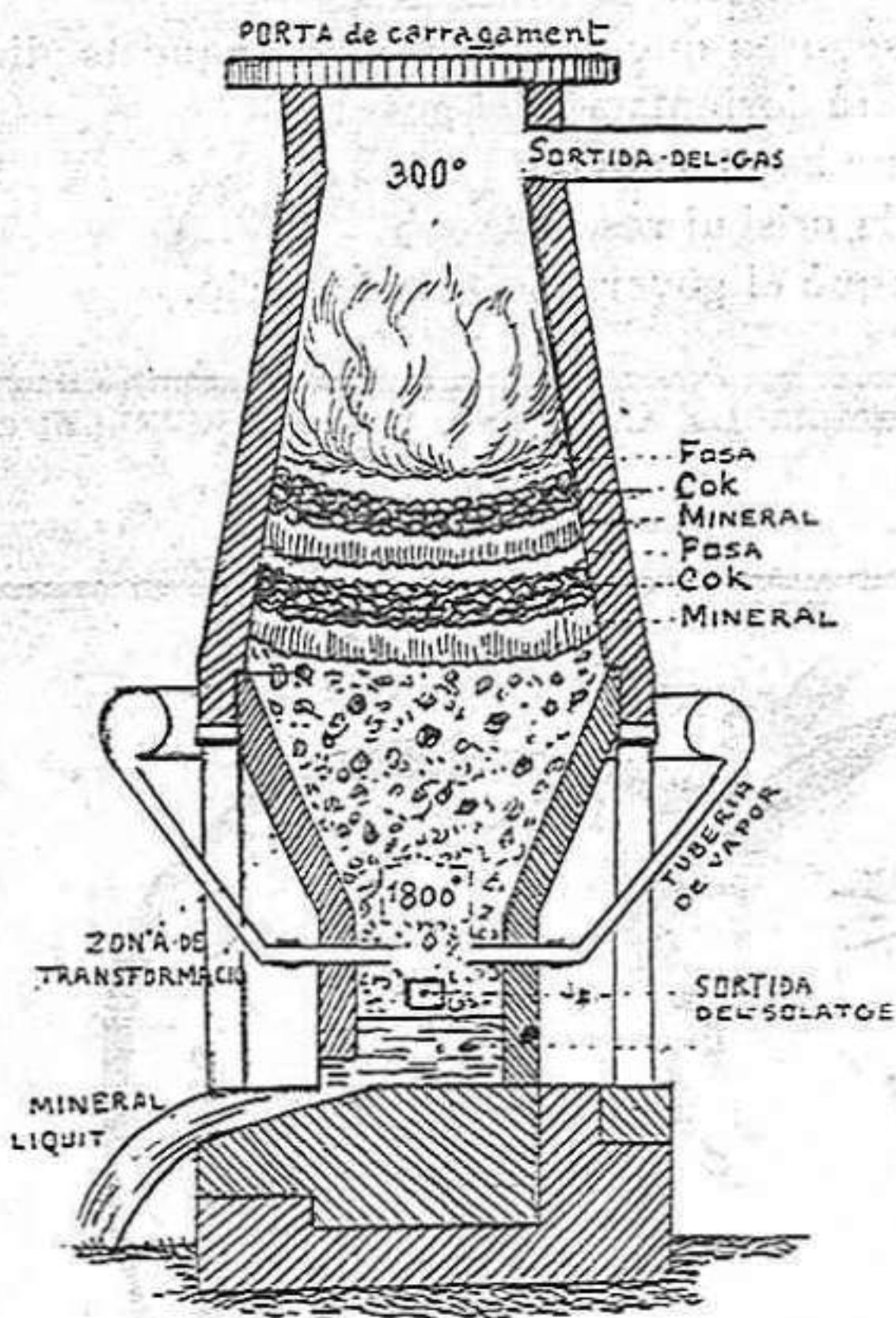
Nou sistema de fosa empleat en l'indústria metalúrgica francesa
