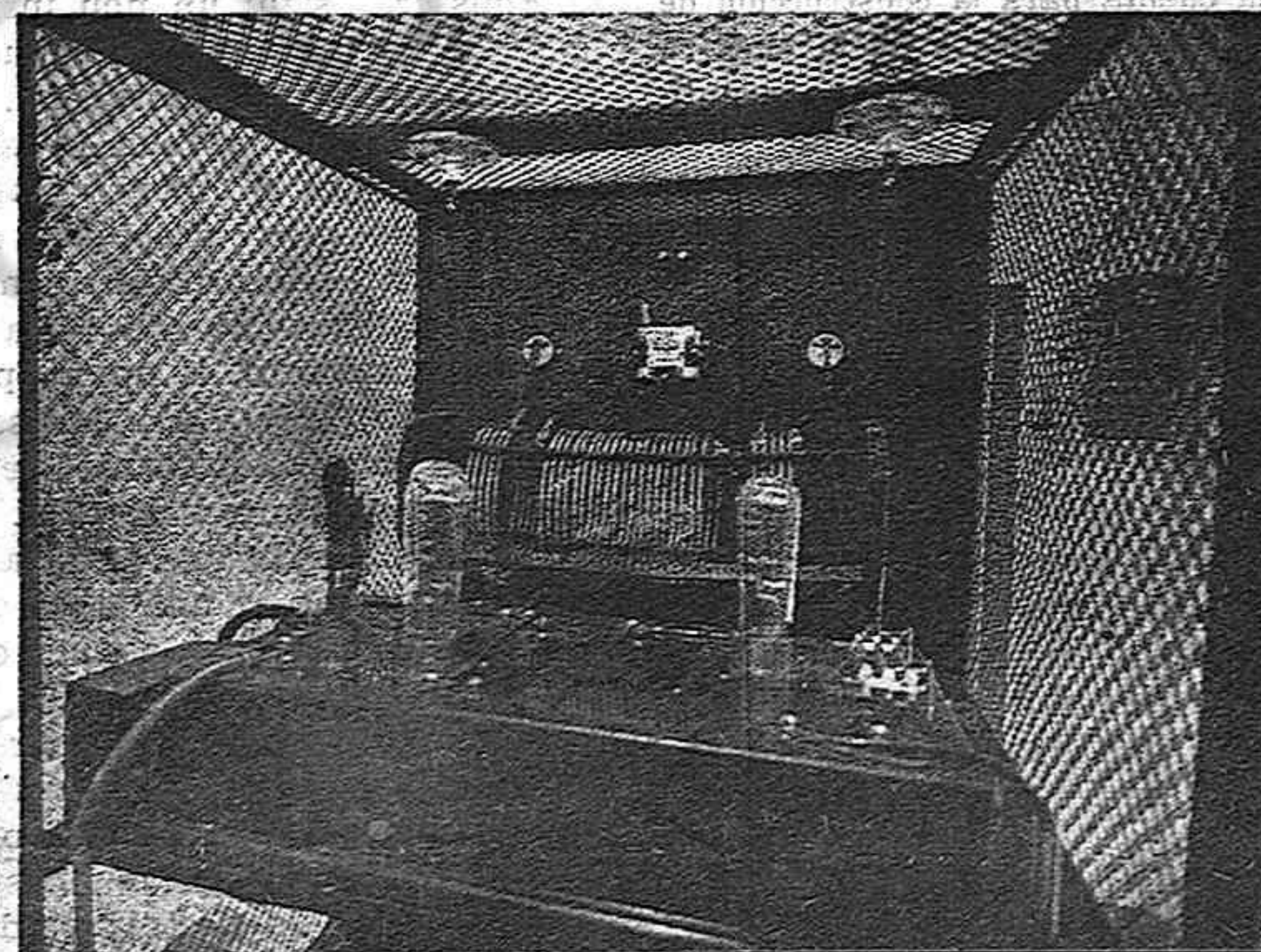
Vista parcial del Amplificador modulado
