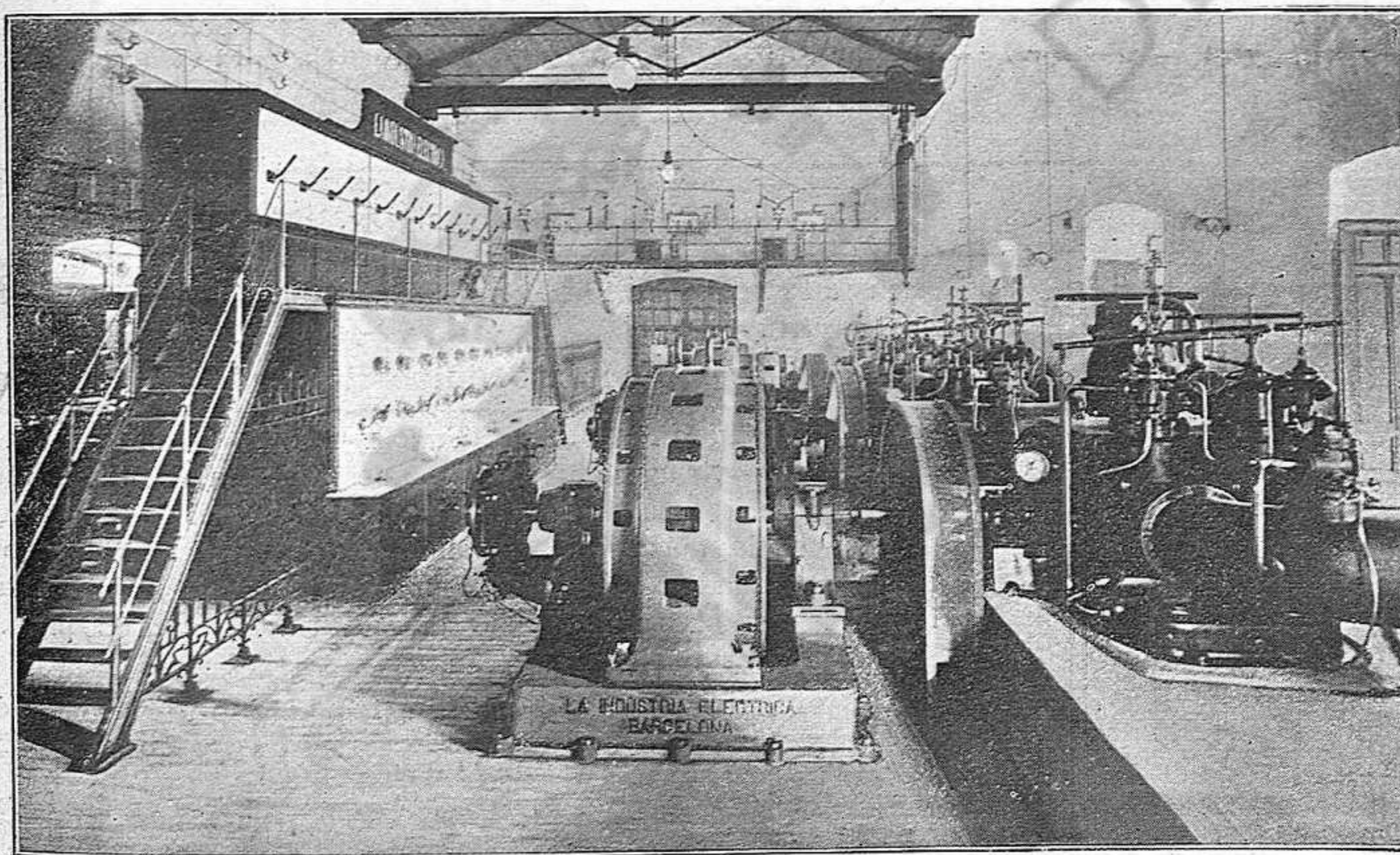
Central de Colmenar Viejo (Santillana), instalada por «La Industria Eléctrica»
