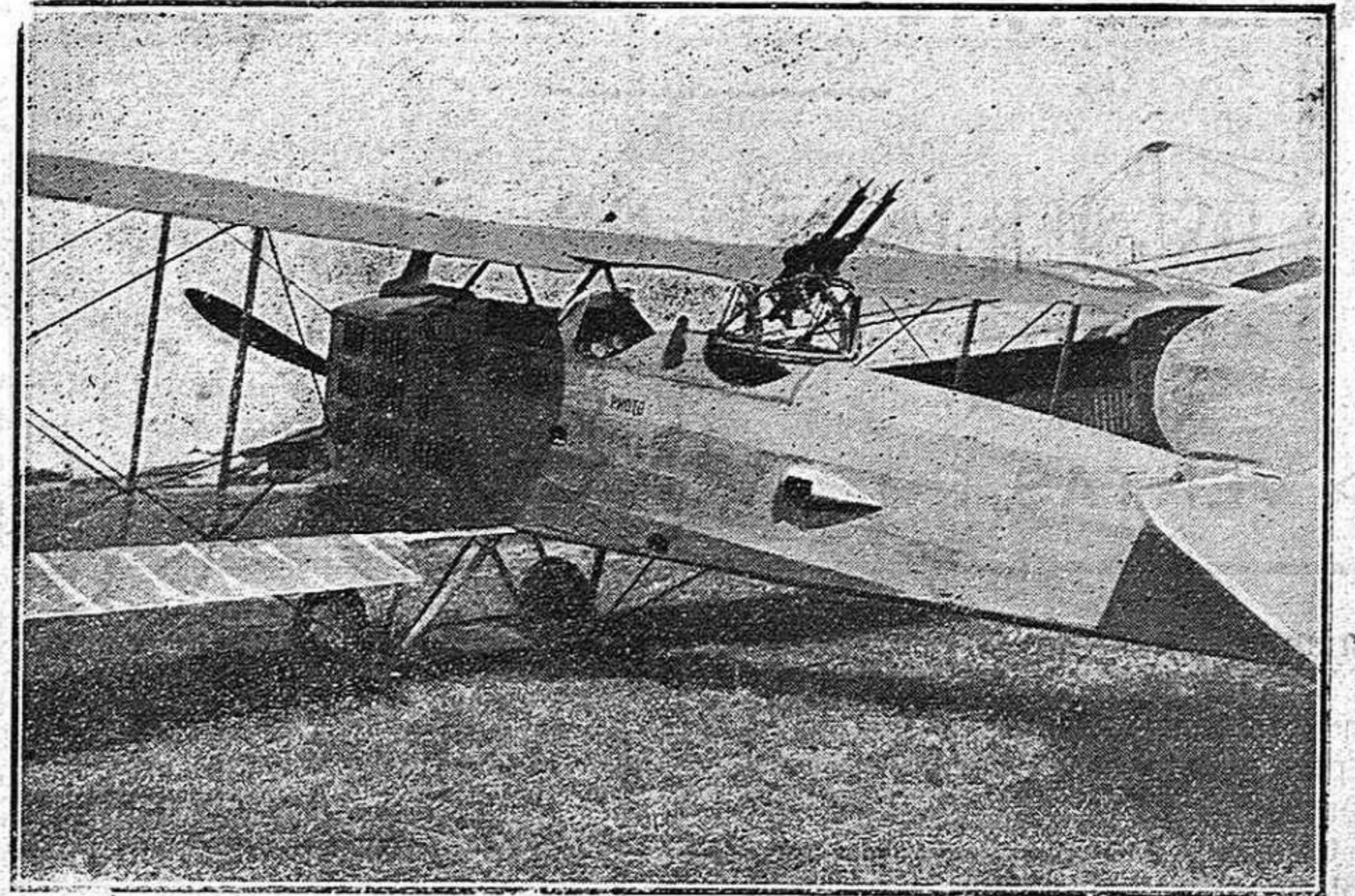
Detalle del avión de bombardeo adquirido, tipo Breguet-Fiat. Además de las ametralladoras de defensa, puede transportar 250 kilogramos de explosivos, para arrojarlos en cada viaje.
