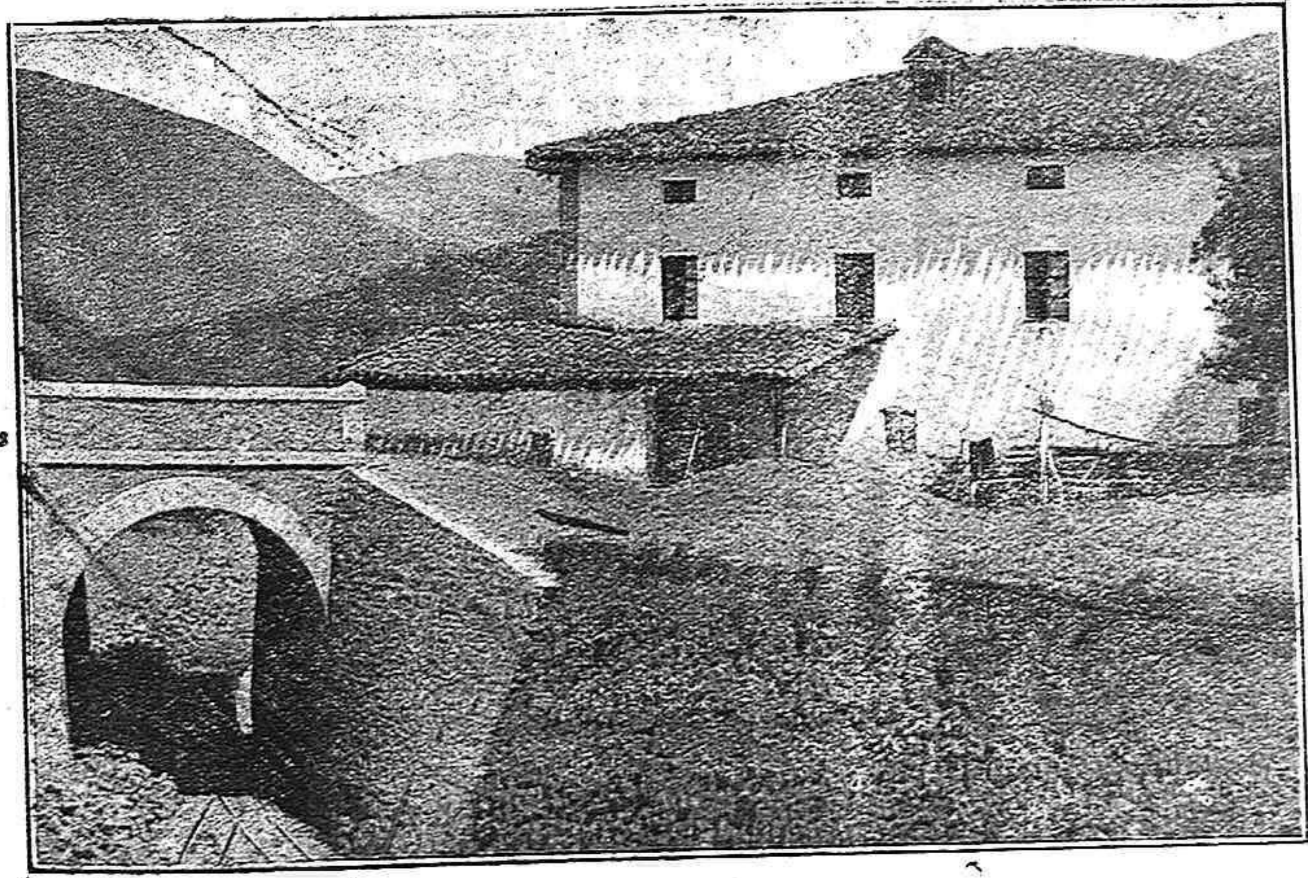
Zubillaga.—Paso superior sobre la vía para tres caminos vecinales
