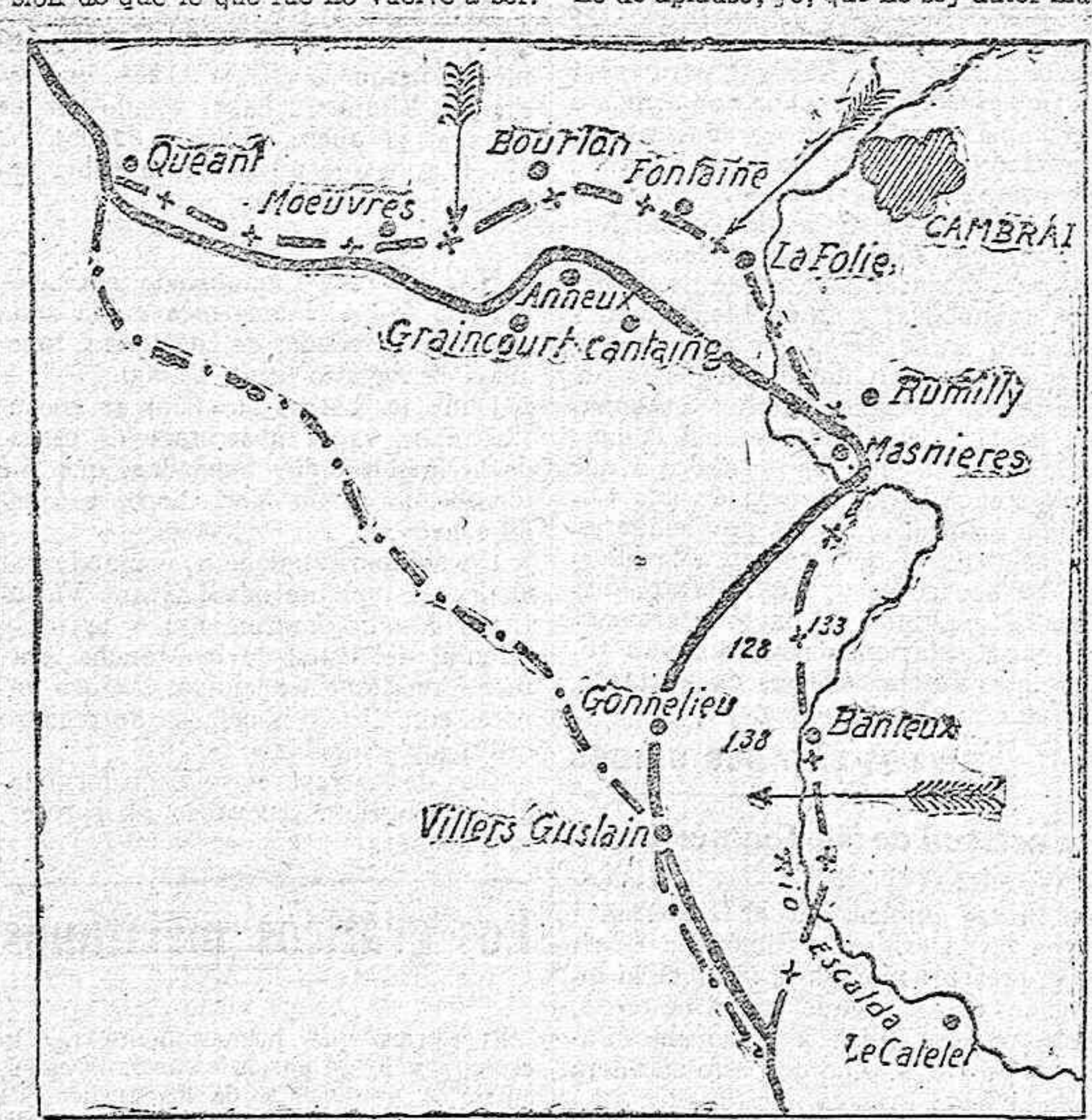
Escala 0 5 10 15 Kilometros. Posición que ocupaban los alemanes el 20 de Noviembre. Posición que tenían el 30 de Noviembre. Posición aproximada actual. Direcciones de ataque.
