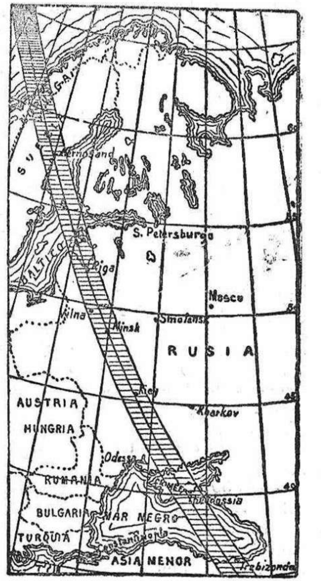
Gráfico del trayecto del cono de sombra que la Luna proyecta sobre los puntos de Europa en que el eclipse de hoy fué total.
