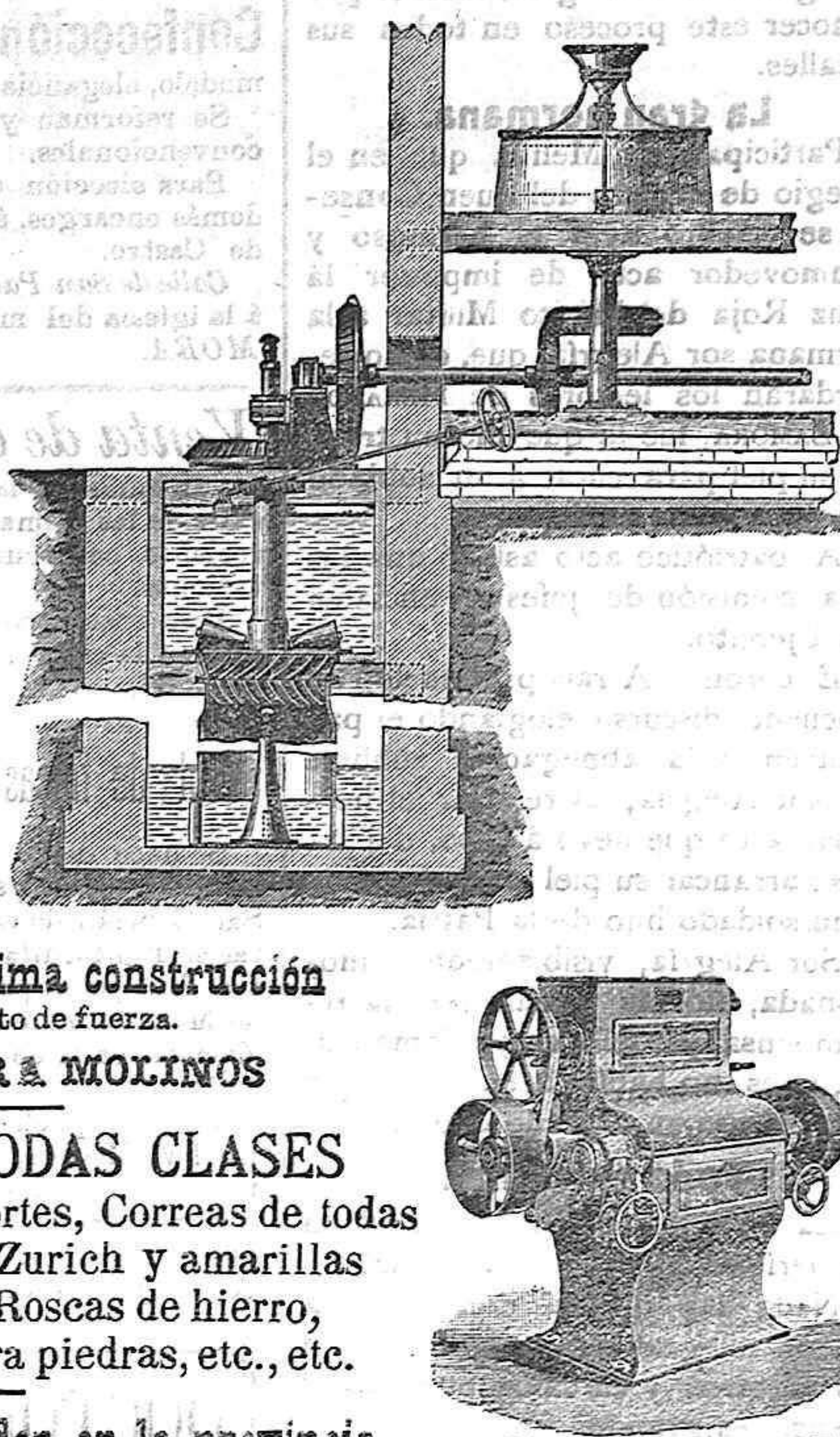
Molino de cilindros
