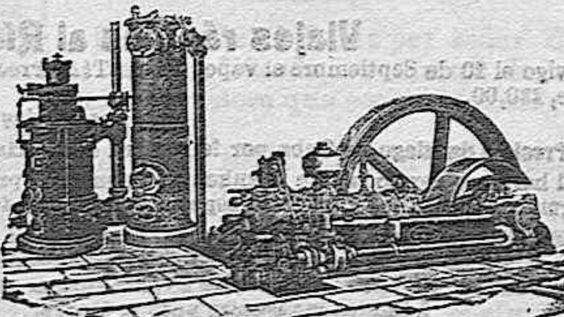
Motor de gas pobre por aspiración «Tangyes».
